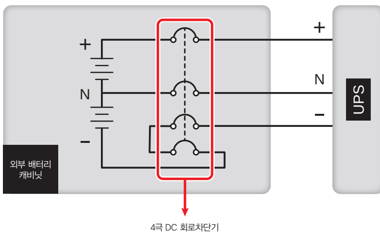
(Figure 6-22: 4극 DC 회로차단기의 설치)
