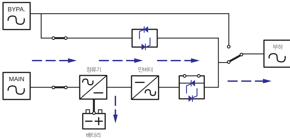
(Figure 4-6: 컨버터 모드 시 UPS의 전력 경로)
