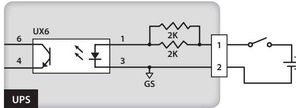
(Figure 5-8: REPO 포트의 구성)
