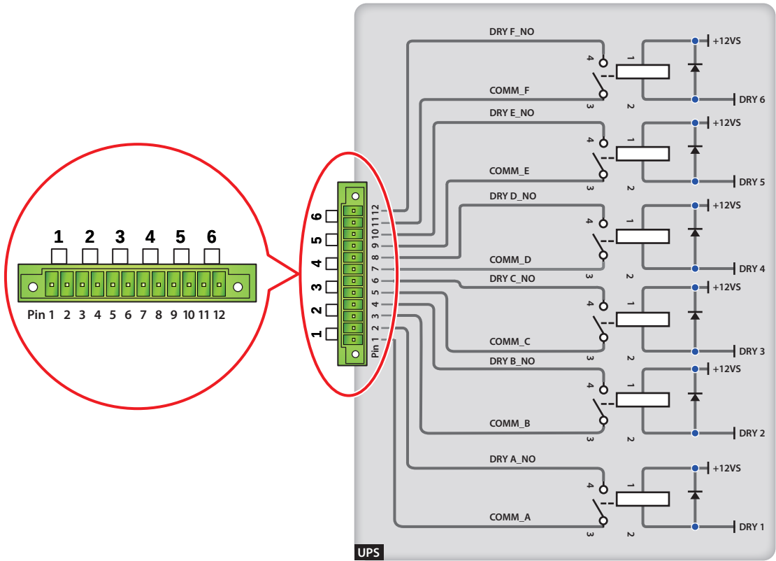
(Figure 5-4: 출력 건식 접점: 핀 구조 및 설계)
