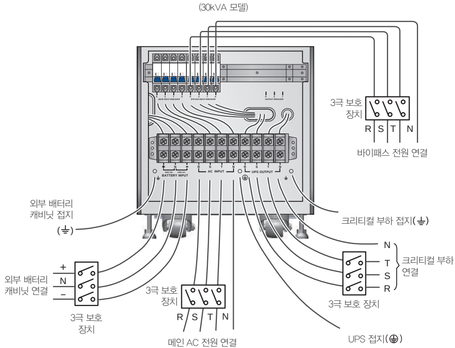
(Figure 6-14: 30kVA UPS 싱글 유닛 듀얼 입력 배선도 I)
