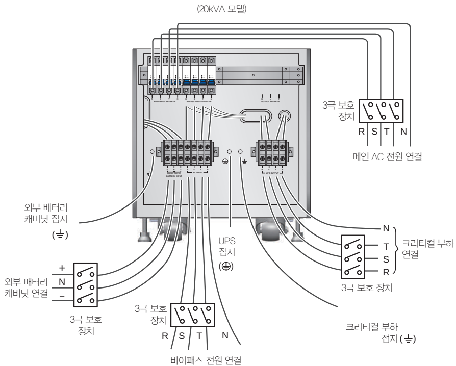
(Figure 6-13: 20kVA UPS 싱글 유닛 듀얼 입력 배선도 II)
