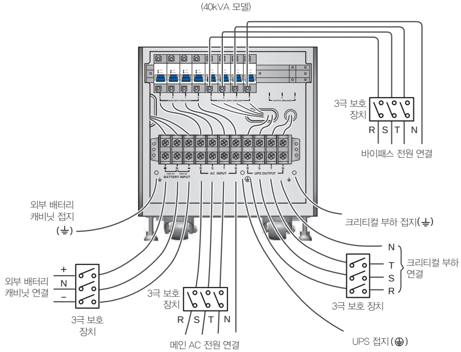
(Figure 6-16: 40kVA UPS 싱글 유닛 듀얼 입력 배선도 I)
