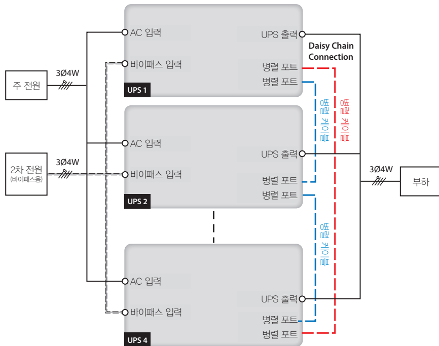
(Figure 6-19: 병렬 유닛 듀얼 입력 배선도)
