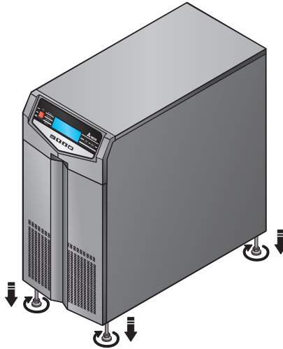
(Figure 6-1: 수평 고정 다리를 이용한 UPS의 안정화)
