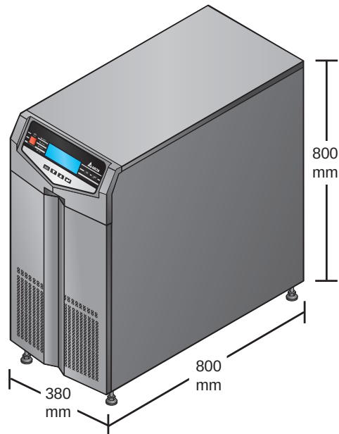
(Figure 3-1: 20/30/40kVA UPS의 외양 및 치수)
