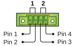
(Figure 5-5: 입력 건식 접점)
