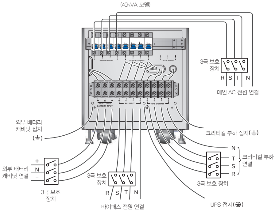
(Figure 6-17: 40kVA UPS 싱글 유닛 듀얼 입력 배선도 II)
