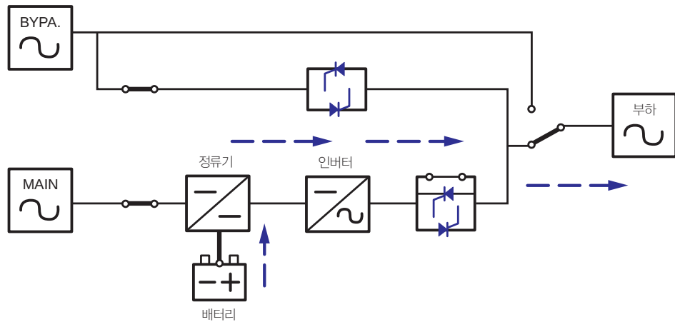
(Figure 4-4: 배터리 모드 시 UPS의 전력 경로)
