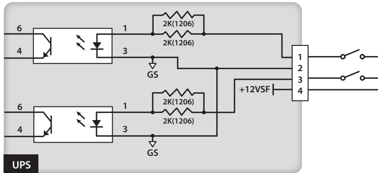
(Figure 5-6: 입력 건식 접점의 구성 I)
