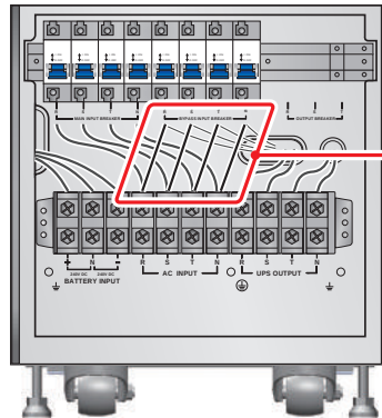
(Figure 6-7: AC 입력 단자 블록과 바 이패스 입력 차단기를 연결하는 4개의 케이블 제거하기)
