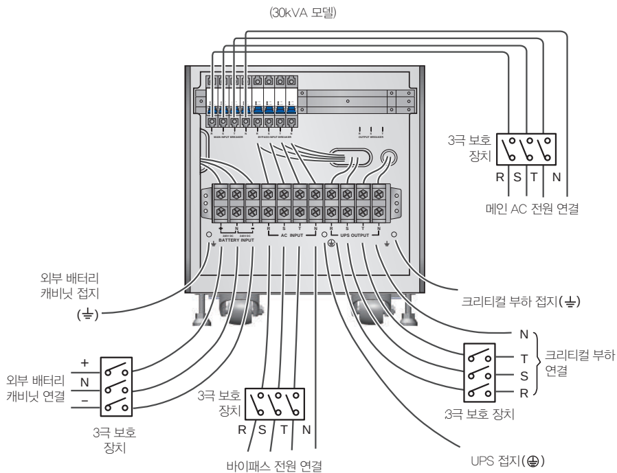
(Figure 6-15: 30kVA UPS 싱글 유닛 듀얼 입력 배선도 II)
