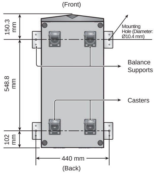
(Figure 6-2: 장착 구멍의 위치)
