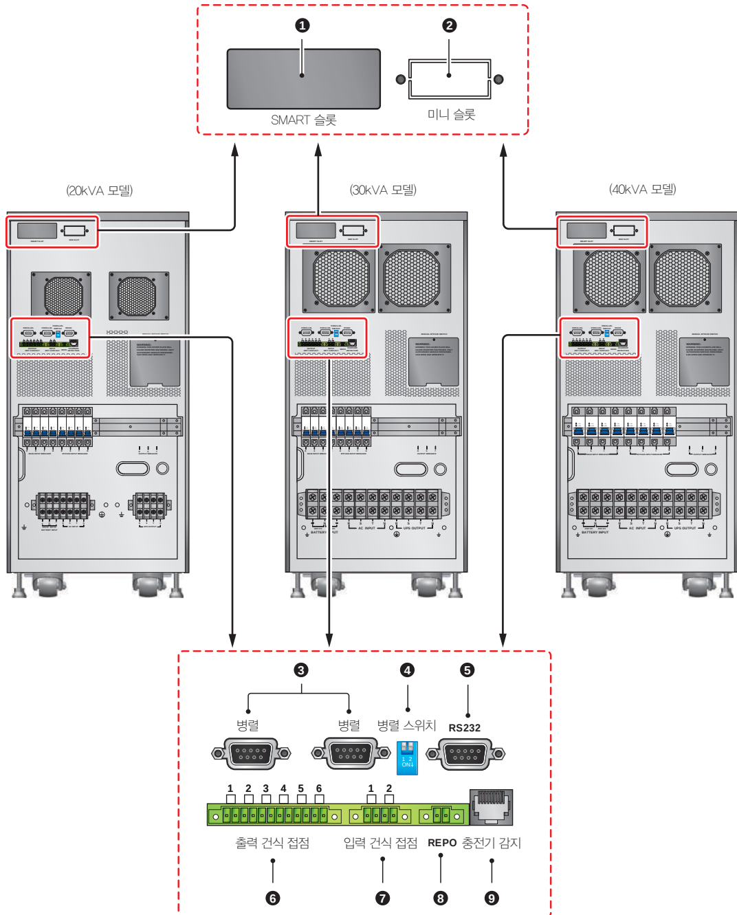
(Figure 5-1: 커뮤니케이션 인터페이스)
