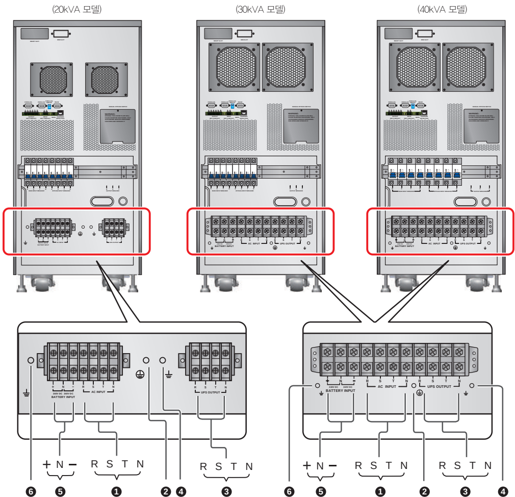
(Figure 6-8: 배선 단자 블록)
