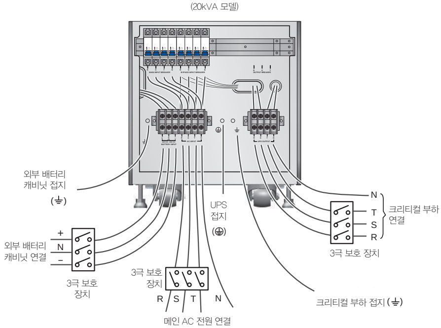
(Figure 6-9: 20kVA UPS 싱글 유닛 싱글 입력 배선도)
