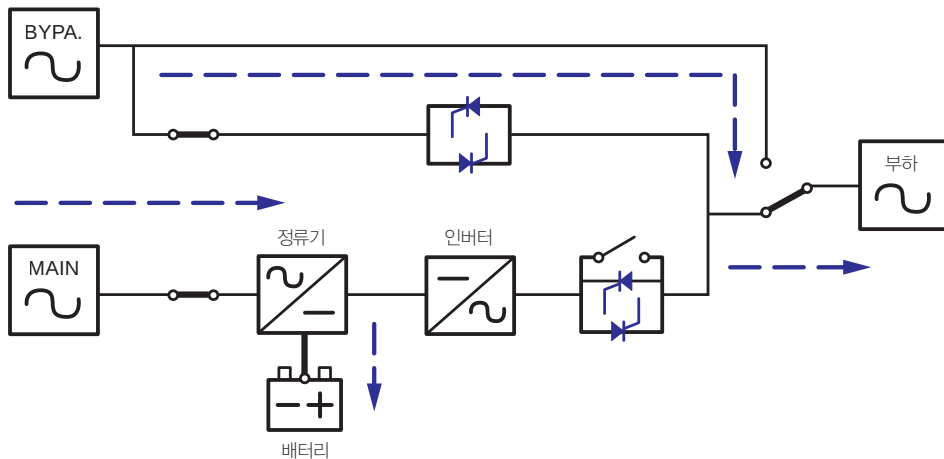
(Figure 4-5: 바이패스 모드 시 UPS의 전력 경로)
