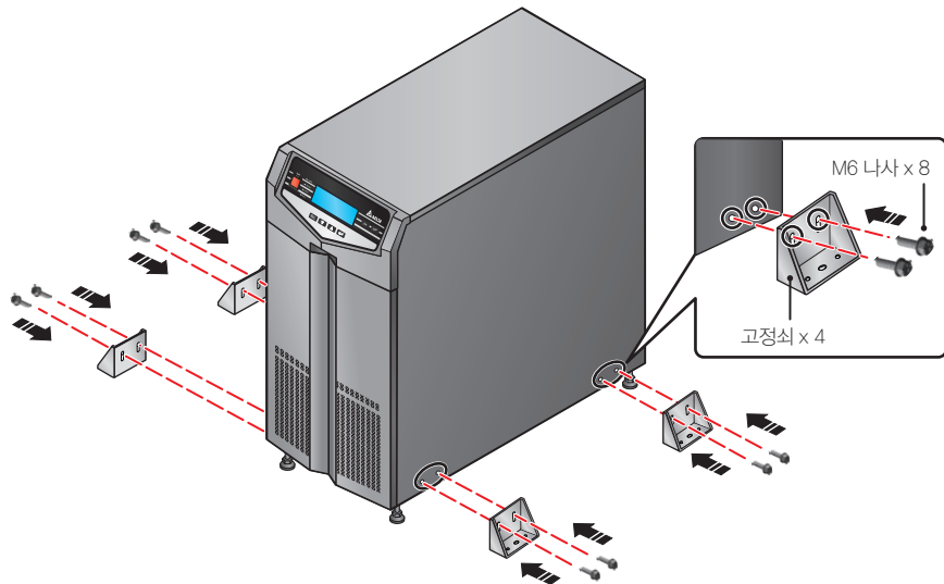
(Figure 6-3: 고정쇠의 설치)
