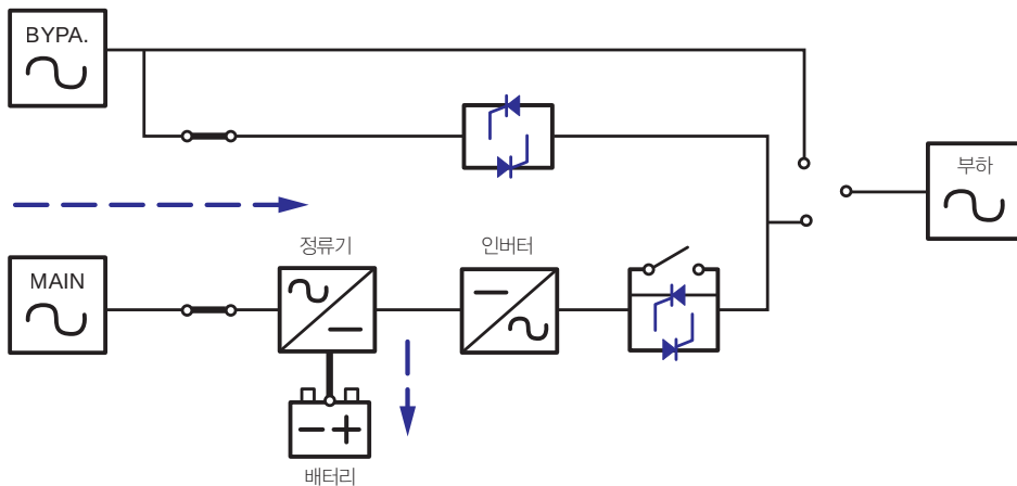
(Figure 4-2: 스탠바이 모드 시 UPS의 전력 경로)
