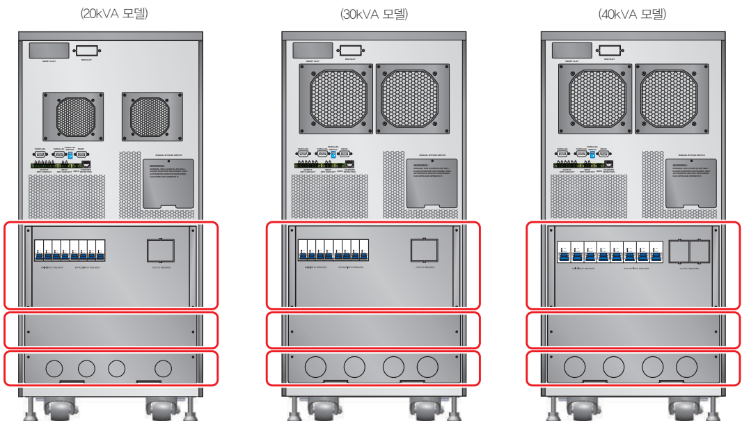
(Figure 6-5: 패널의 위치)
