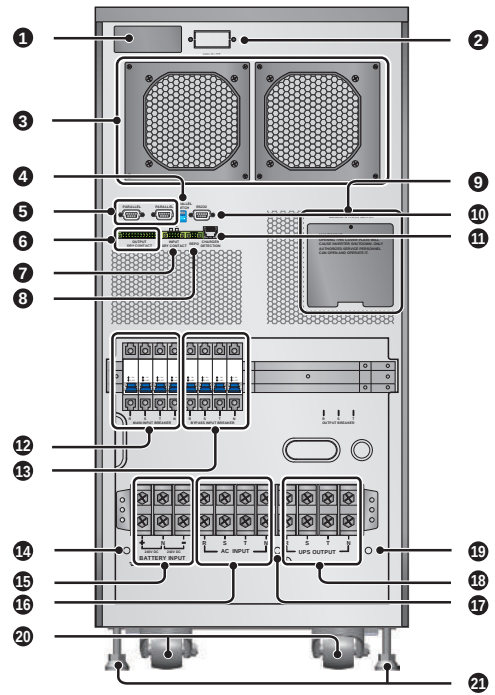
(Figure 3-4: 30kVA 리어 패널)
