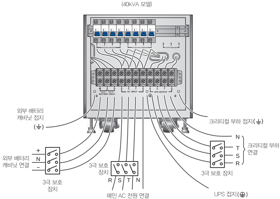
(Figure 6-11: 40kVA UPS 싱글 유닛 싱글 입력 배선도)
