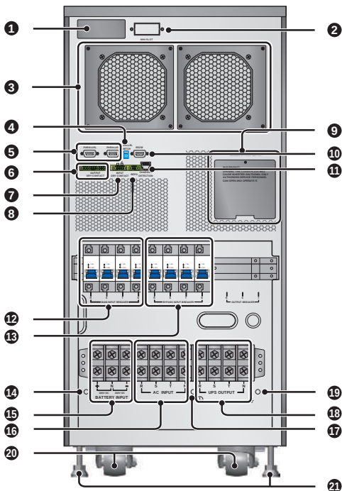
(Figure 3-5: 40kVA 리어 패널)
