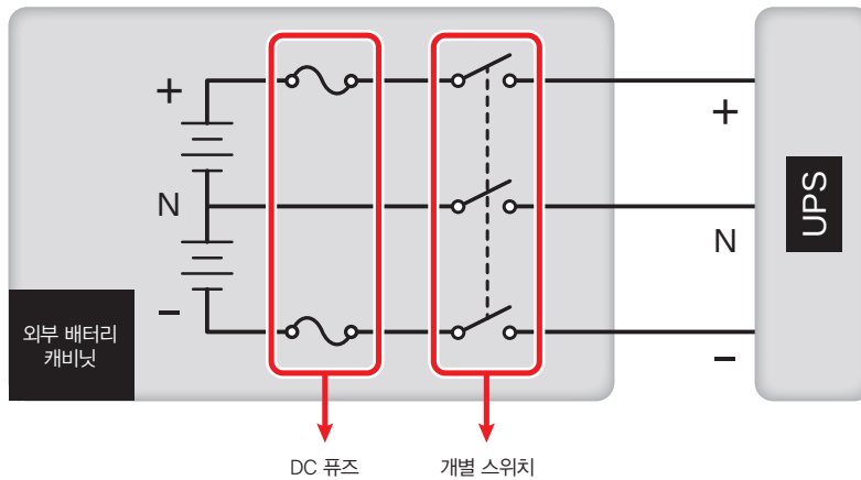
(Figure 6-21: DC 퓨즈와 직렬 연결된 독립 스위치의 설치)
