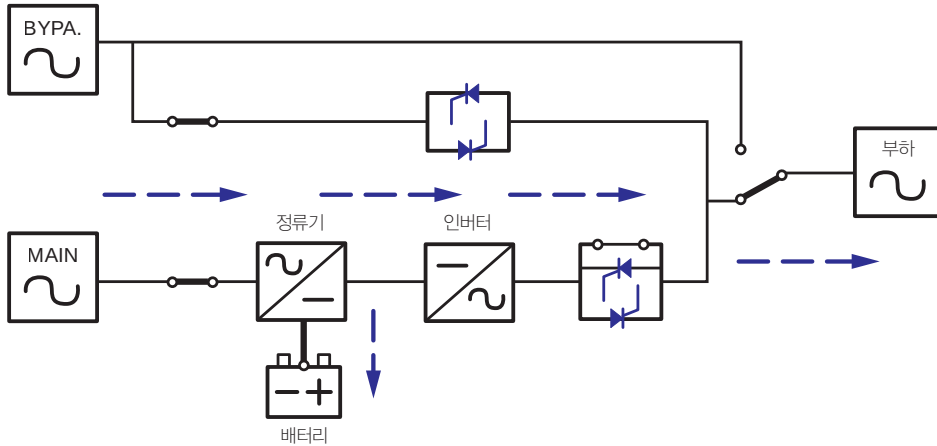
(Figure 4-1: 온라인 모드 시 UPS의 전력 경로)
