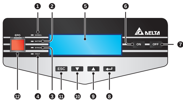
(Figure 3-2: 프론트 패널)
