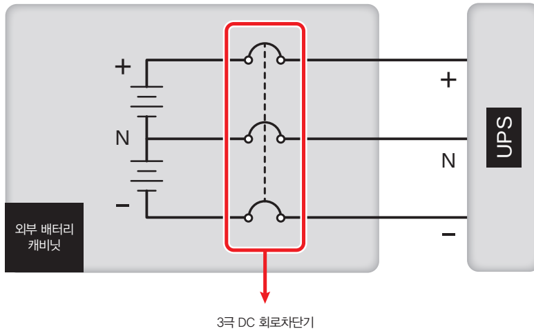
(Figure 6-23: 3극 DC 회로차단기의 설치)
