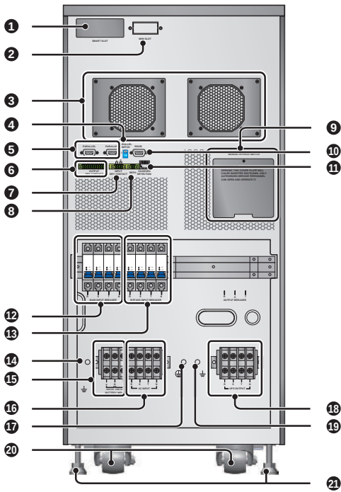
(Figure 3-3: 20kVA 리어 패널)
