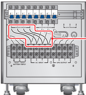
(Figure 6-6: AC 입력 단자 블록과 메인 입력 차단기를 연결하는 4개의 케이블 제거하기)
