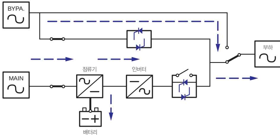
(Figure 4-3: ECO 모드 시 UPS의 전력 경로)
