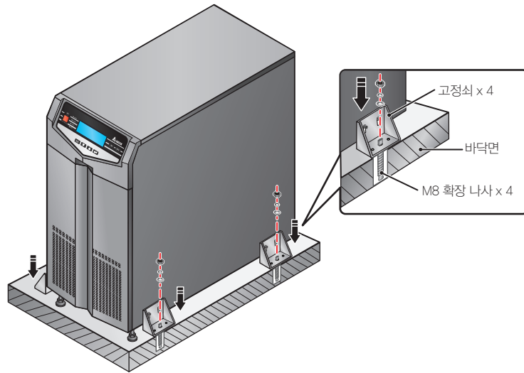
(Figure 6-4: 고정쇠의 바닥면 고정)
