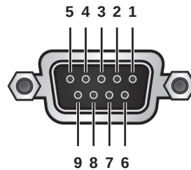
(Figure 5-3: RS232 포트)
