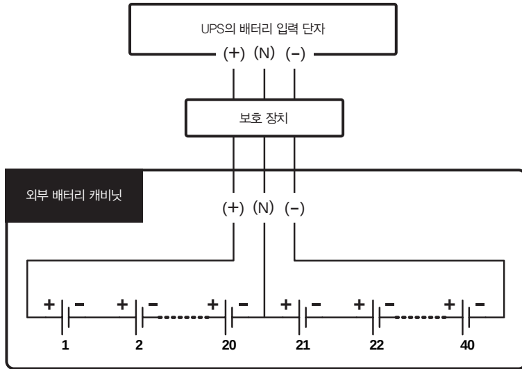
(Figure 6-20: 외부 배터리 캐비닛의 연결)
