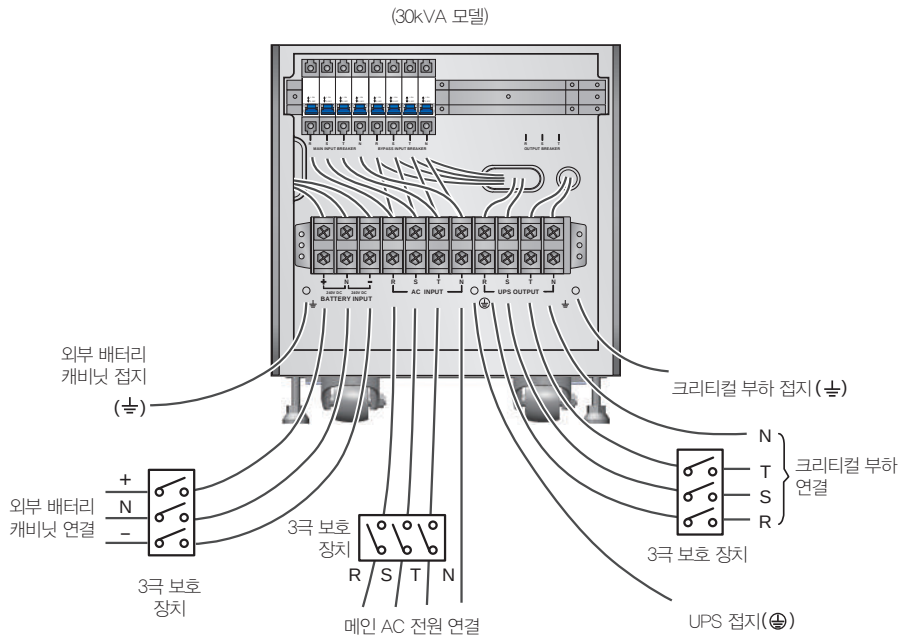
(Figure 6-10: 30kVA UPS 싱글 유닛 싱글 입력 배선도)
