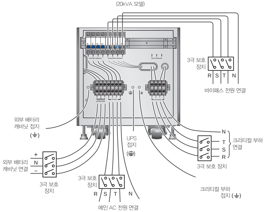
(Figure 6-12: 20kVA UPS 싱글 유닛 듀얼 입력 배선도 I)
