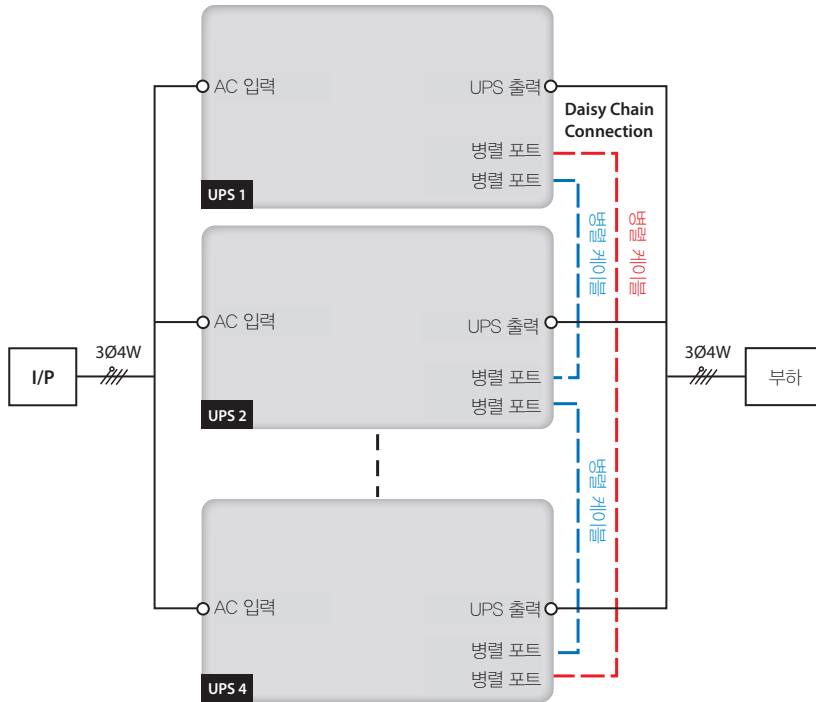
(Figure 6-18: 병렬 유닛 싱글 입력 배선도)
