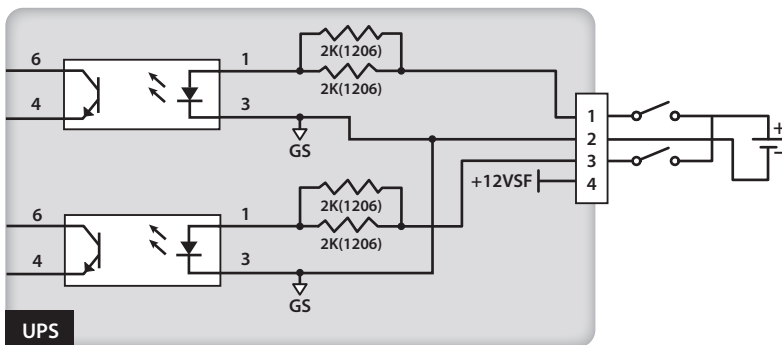
(Figure 5-7: 입력 건식 접점의 구성 II)
