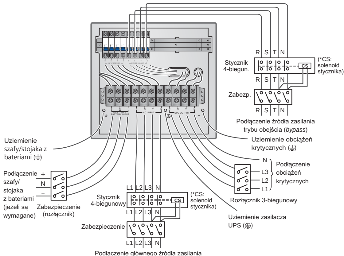
(Rysunek 6-15: Schemat okablowania w trybie pojedynczej jednostki i podwójnego źródła zasilania dla modelu o mocy 30 kVA)
