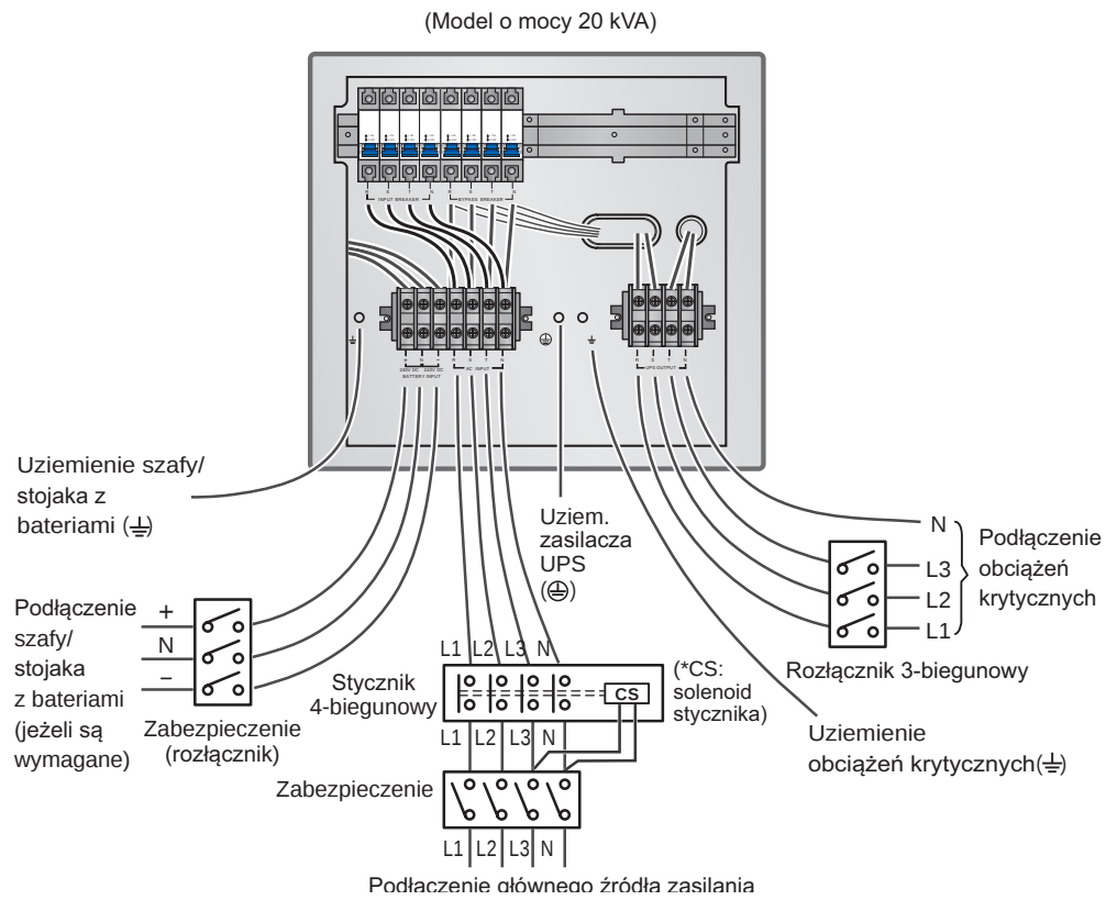
(Rysunek 6-10: Schemat okablowania w trybie pojedynczej jednostki i pojedynczego źródła zasilania dla modelu o mocy 20 kVA)
