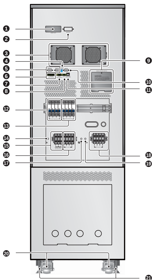
(Rysunek 3-6: Panel tylny modelu o mocy 20 kVA)
