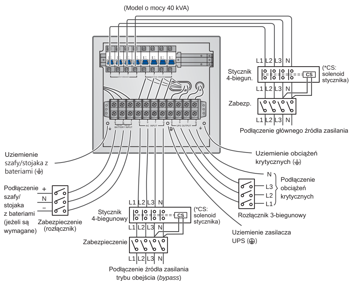
(Rysunek 6-18: Schemat okablowania w trybie pojedynczej jednostki i podwójnego źródła zasilania dla modelu o mocy 40 kVA - sposób II)
