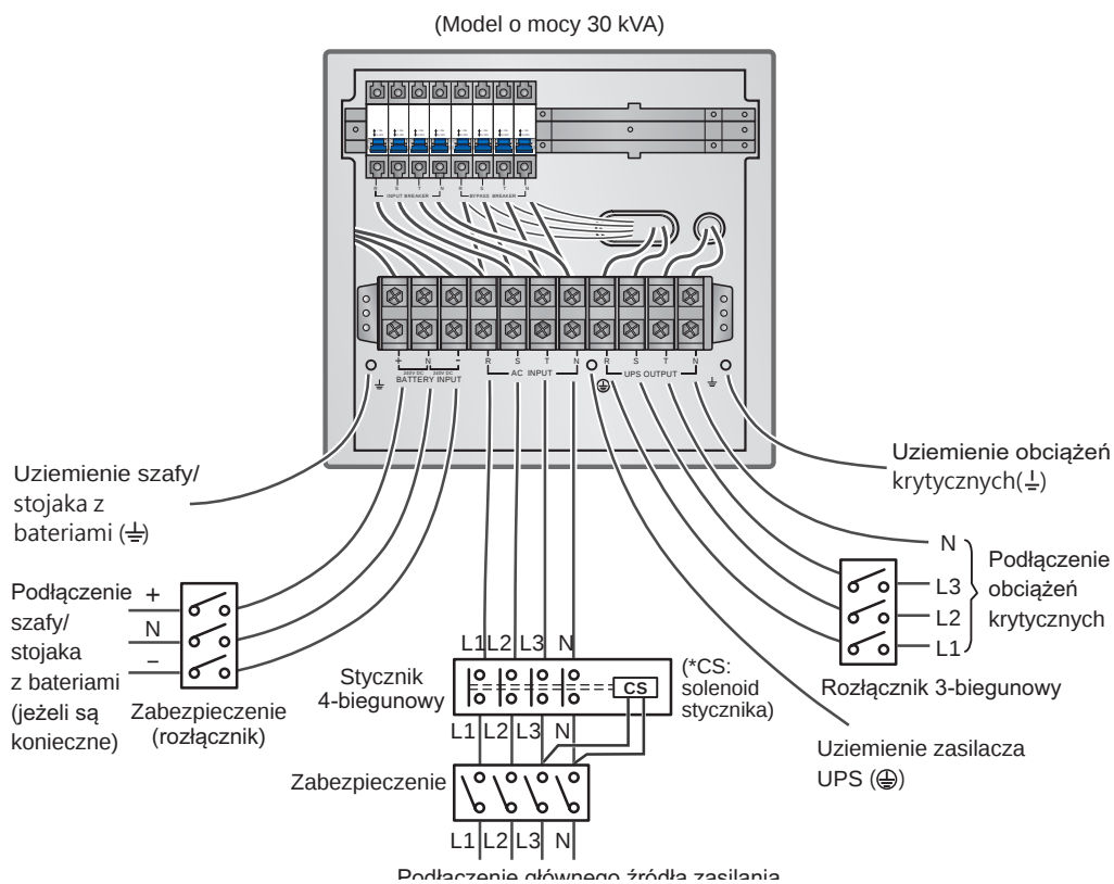
(Rysunek 6-11: Schemat okablowania w trybie pojedynczej jednostki i pojedynczego źródła zasilania dla modelu o mocy 30 kVA)
