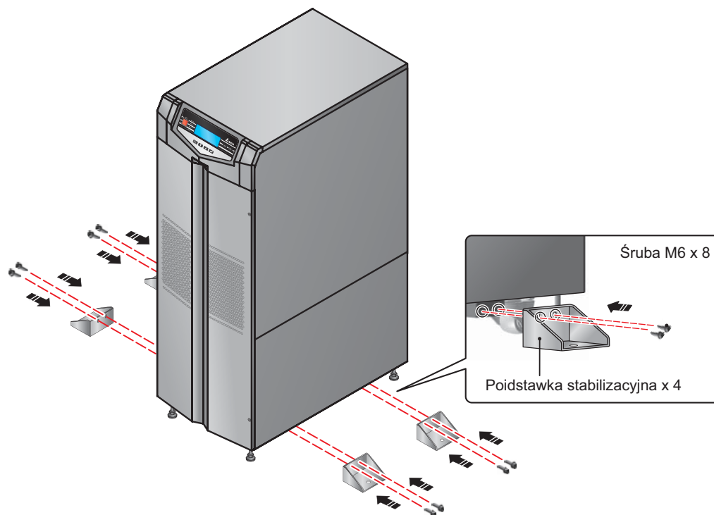
(Rysunek 6-3: Montaż podstawek stabilizacyjnych)
