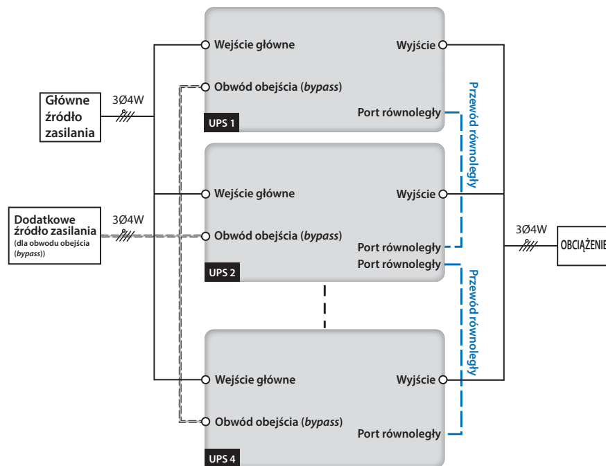
(Rysunek 6-20: Schemat okablowania w trybie jednostek równoległych i podwójnego źródła zasilania)
