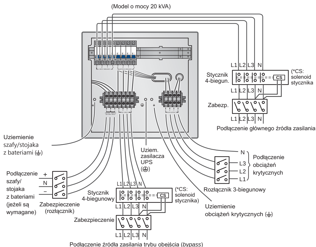
(Rysunek 6-14: Schemat okablowania w trybie pojedynczej jednostki i podwójnego źródła zasilania dla modelu o mocy 20 kVA - sposób II) (Model o mocy 30 kVA)
