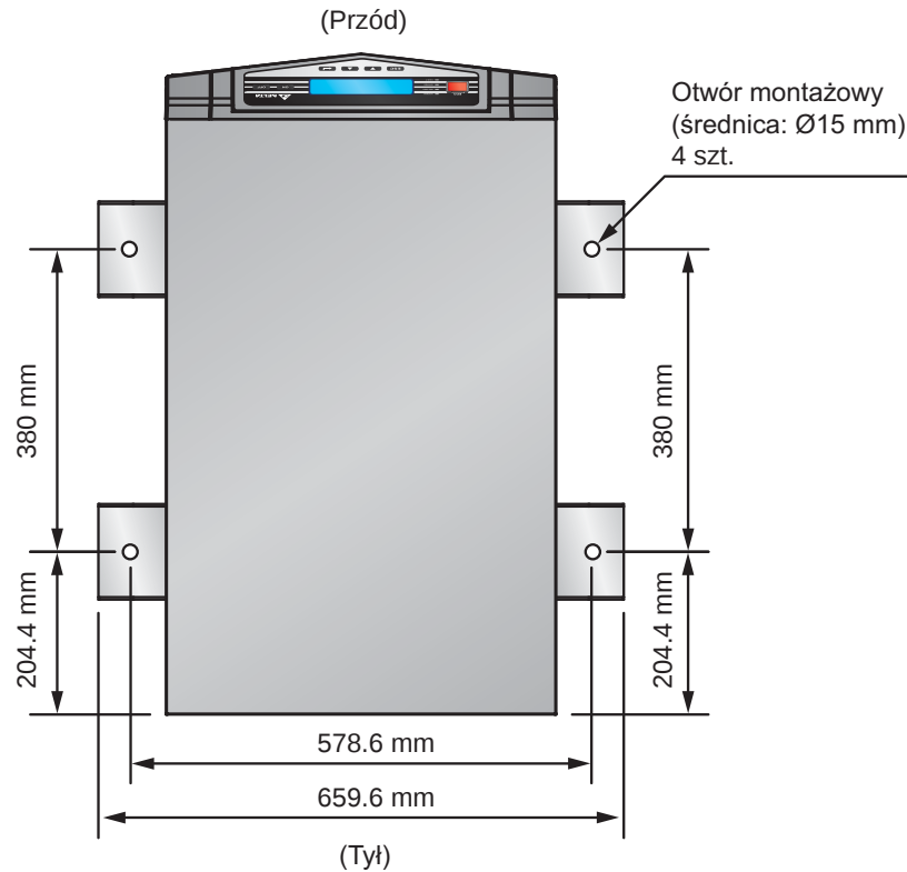
(Rysunek 6-2: Lokalizacja otworów montażowych)
