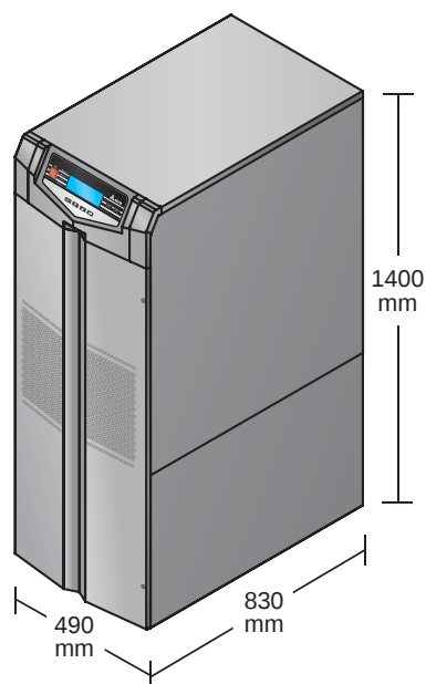
(Rysunek 3-1: 2 Wygląd i wymiary - modele o mocy 20/30/40 kVA)
