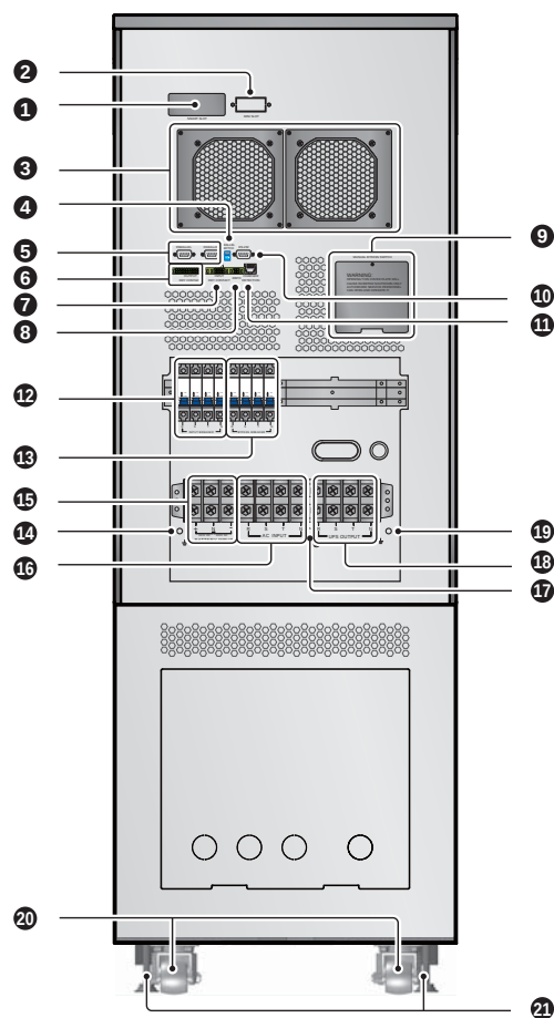
(Rysunek 3-7: Panel tylny modelu o mocy 30 kVA)
