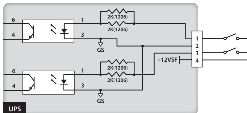
(Rysunek 5-6: Konfiguracja cyfrowych wejść sygnałowych I)
