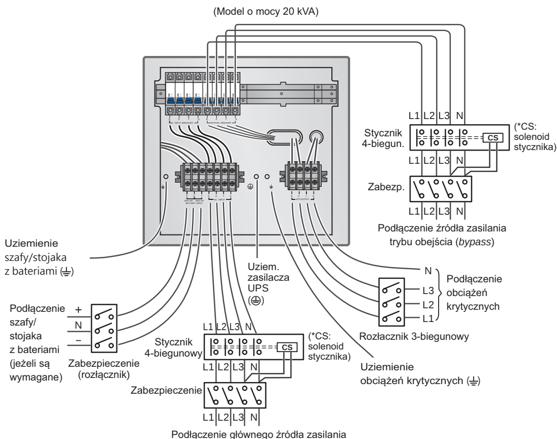
(Rysunek 6-13: Schemat okablowania w trybie pojedynczej jednostki i podwójnego źródła zasilania dla modelu o mocy 20 kVA)
