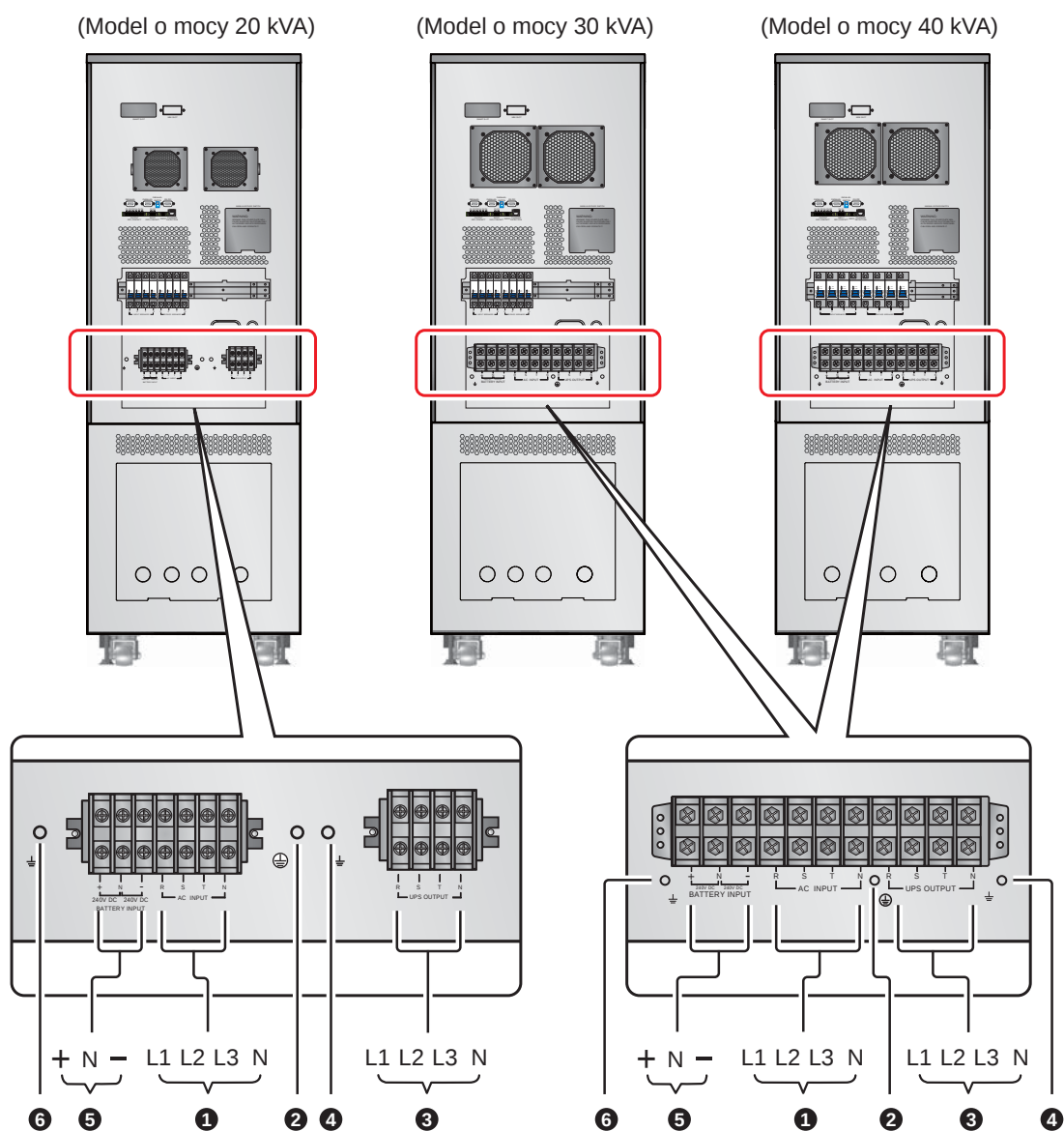
(Rysunek 6-8: Blok podłączeniowy)
