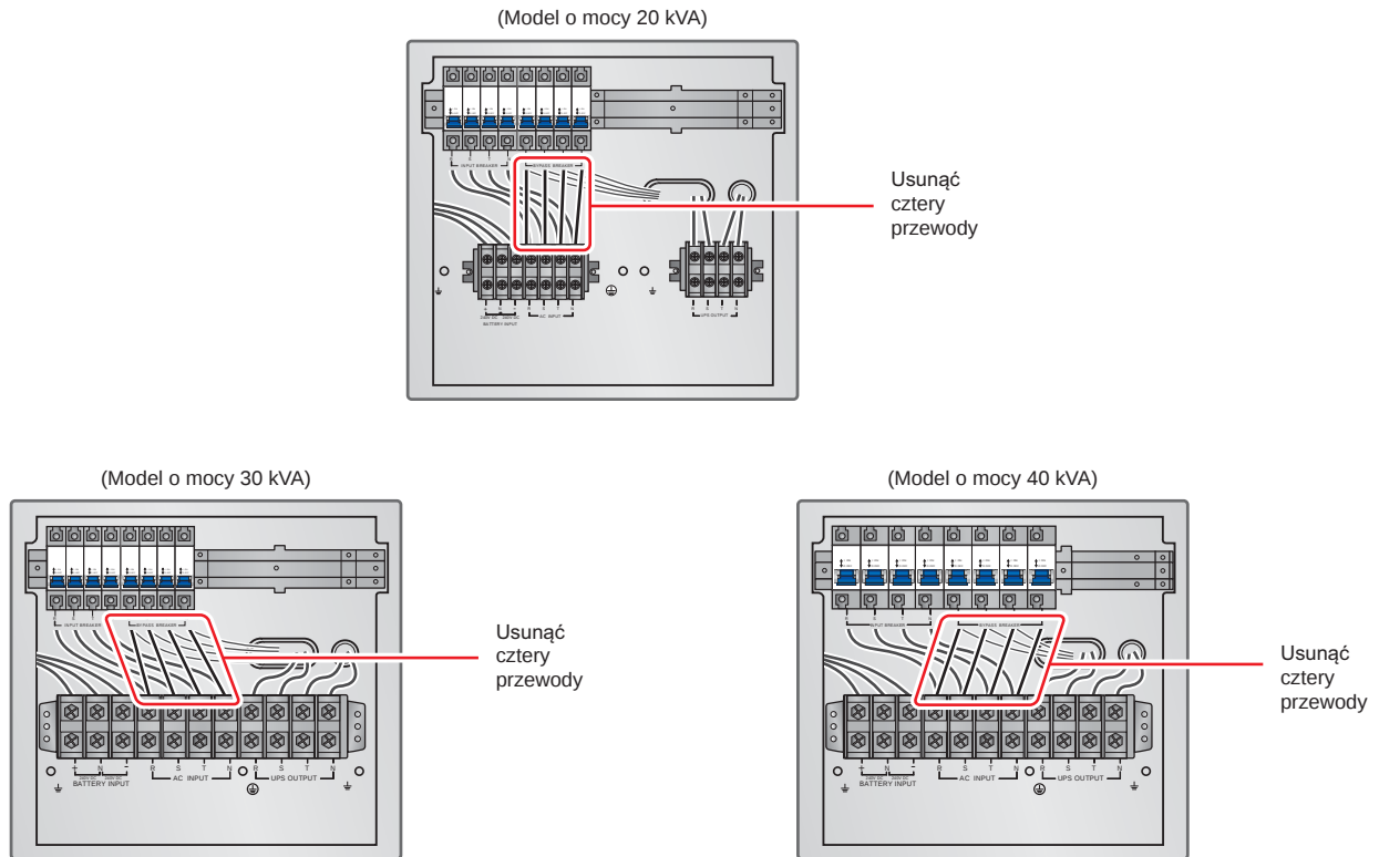
(Rysunek 6-7: Usuwanie czterech przewodów łączących blok podłączeniowy zasilania głównego wyłącznikiem zasilania trybu obejścia ( bypass ))
