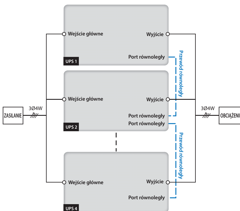
(Rysunek 6-19: Schemat okablowania w trybie jednostek równoległych i pojedynczego źródła zasilania)
