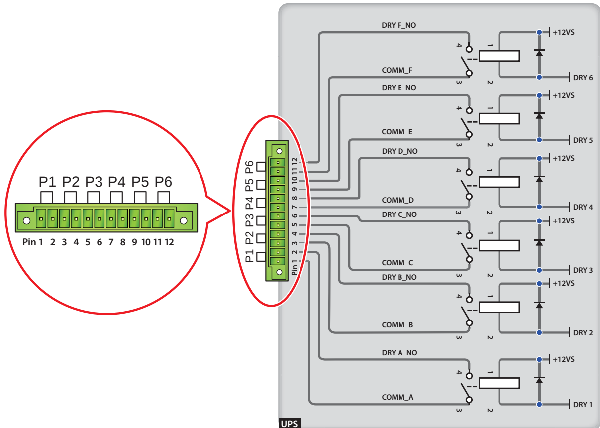
(Rysunek 5-4: Cyfrowe wyjścia sygnałowe: budowa i rozkład PINów)
