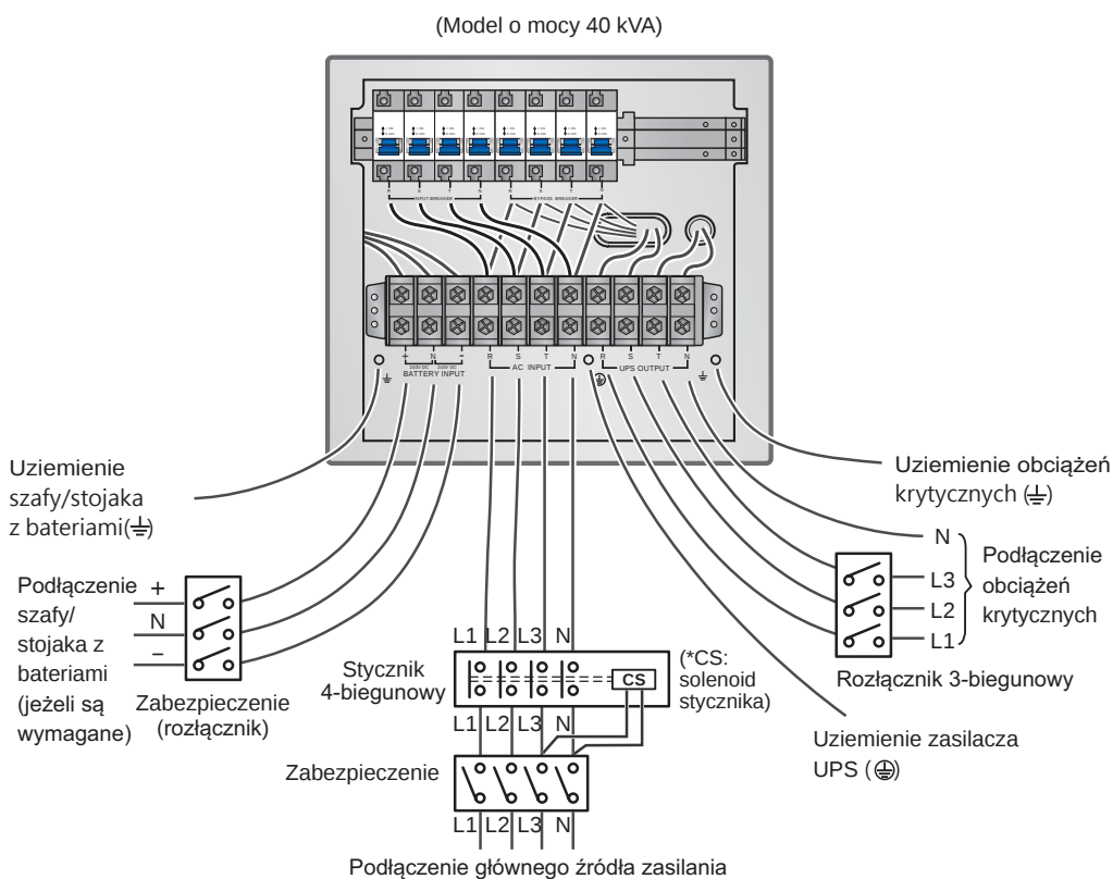
(Rysunek 6-12: Schemat okablowania w trybie pojedynczej jednostki i pojedynczego źródła zasilania dla modelu o mocy 40 kVA)
