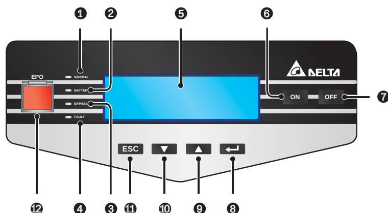
(Rysunek 3-5: Panel sterowania)
