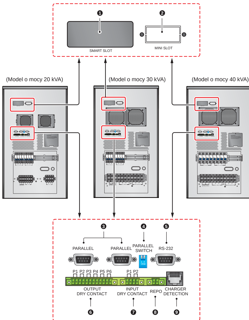
(Rysunek 5-1: Interfejsy komunikacyjne)
