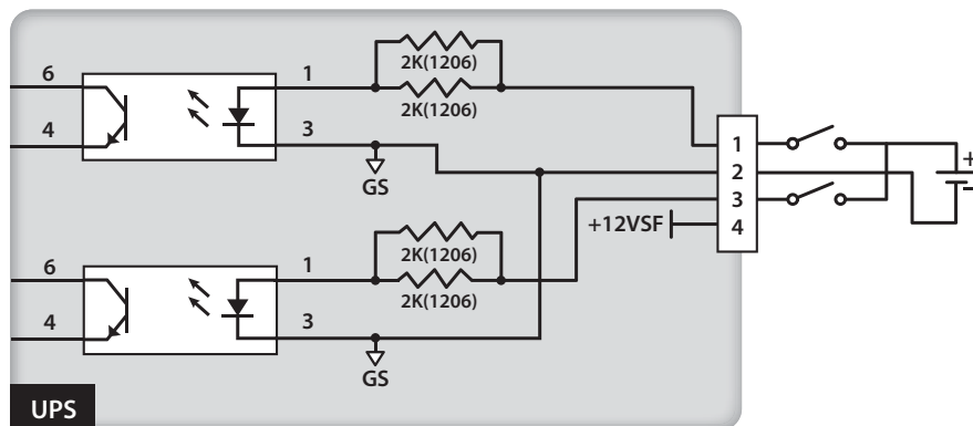
(Rysunek 5-7: Konfiguracja cyfrowych wejść sygnałowych II)
