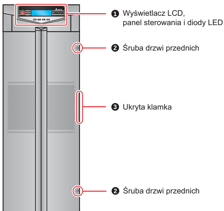
(Rysunek 3-2: Panel przedni)
