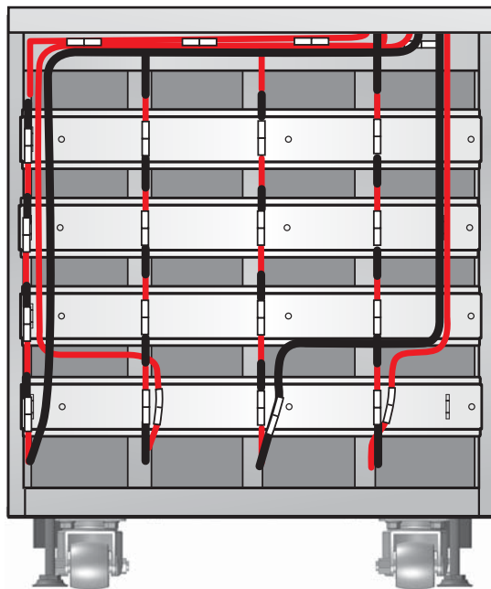
(Rysunek 6-9: Instalacja zestawu bateryjnego)
