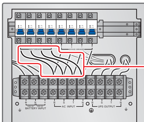
(Rysunek 6-6: Usuwanie czterech przewodów łączących blok podłączeniowy zasilania głównego z głównym wyłącznikiem zasilania)
