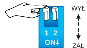
(Rysunek 5-2: Przełącznik ) (trybu portów równoległych)
