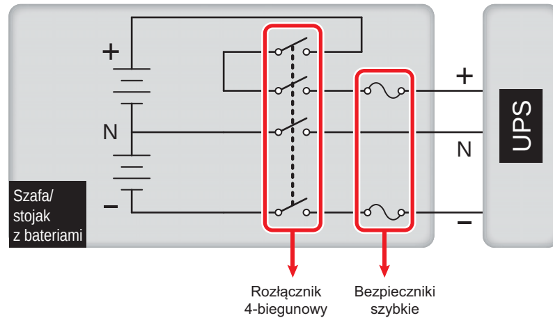
(Rysunek 6-21: Sposób podłączenia 4-biegunowego rozłącznika i bezpieczników szybkich)
