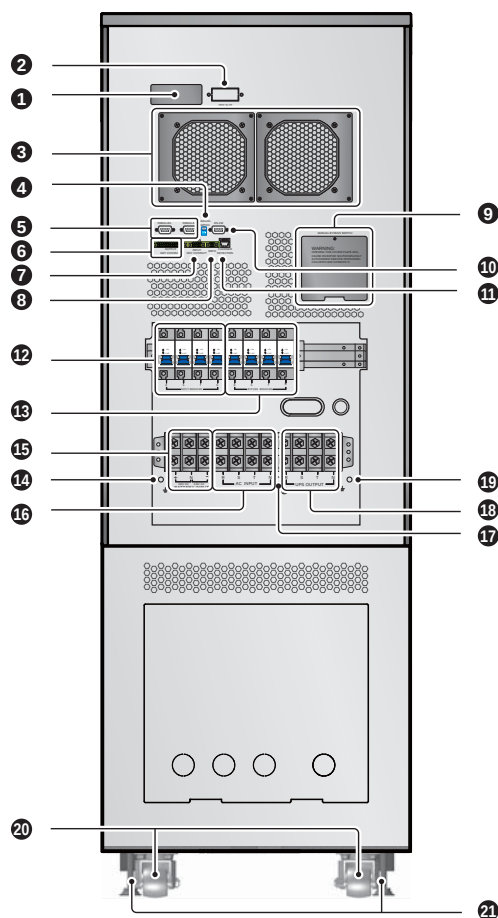
(Rysunek 3-8: Panel tylny modelu o mocy 40 kVA)
