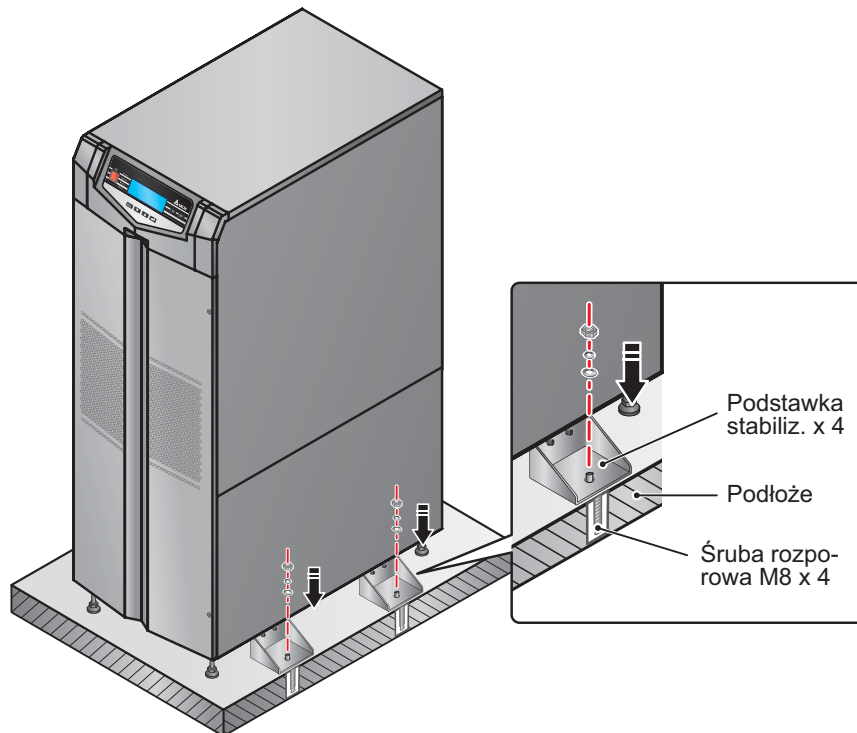
(Rysunek 6-4: Mocowanie podstawek stabilizacyjnych do podłoża)
