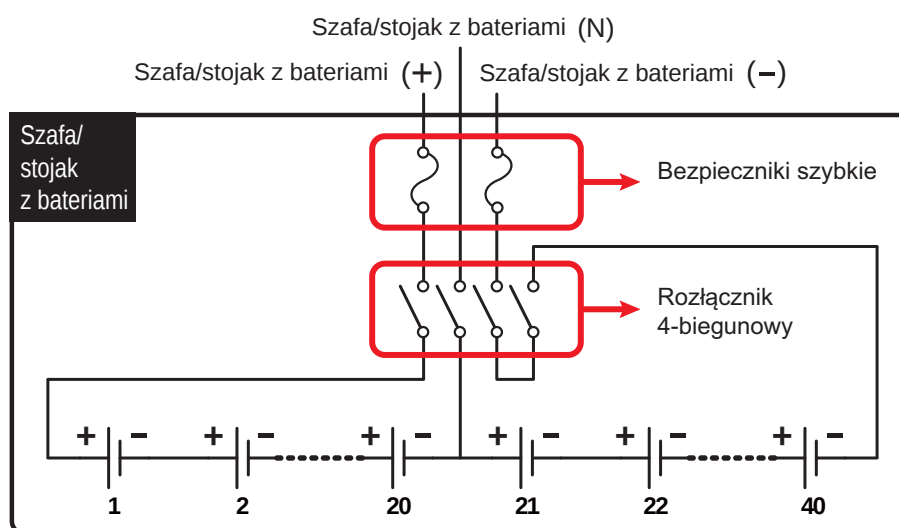
(Rysunek 6-23: Podłączanie zewnętrznej szafy/stojaka z bateriami)
