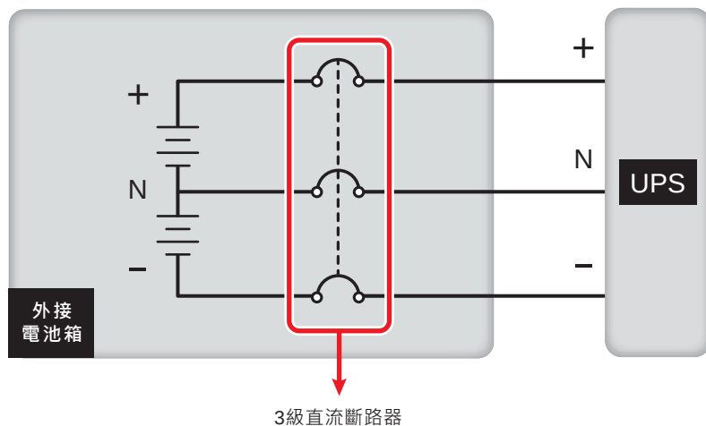
( 圖 5-21：安裝 3 極直流斷路器 )
