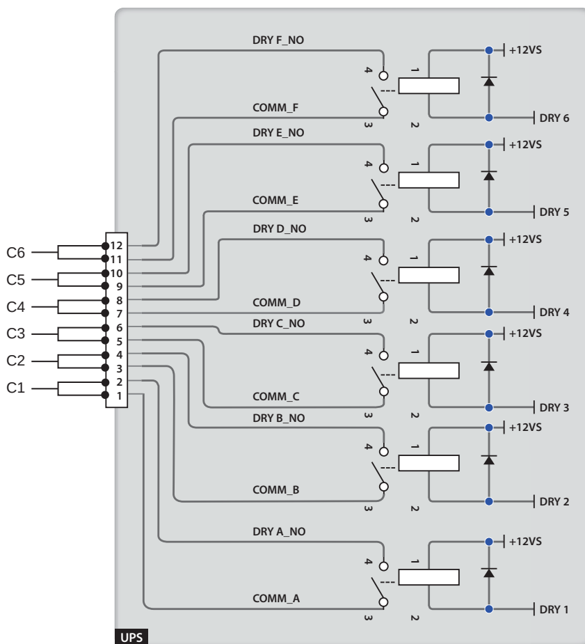
(圖 4-5：輸出乾接點腳位圖)
