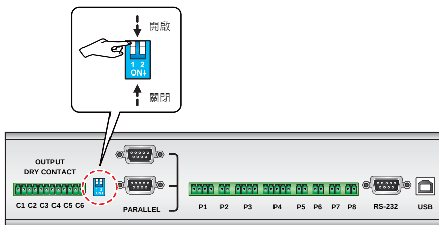
(圖 7-3：設定並聯開關)
