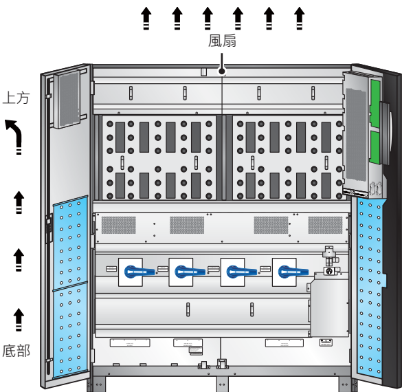
(圖 5-1：風扇送風方向圖)
