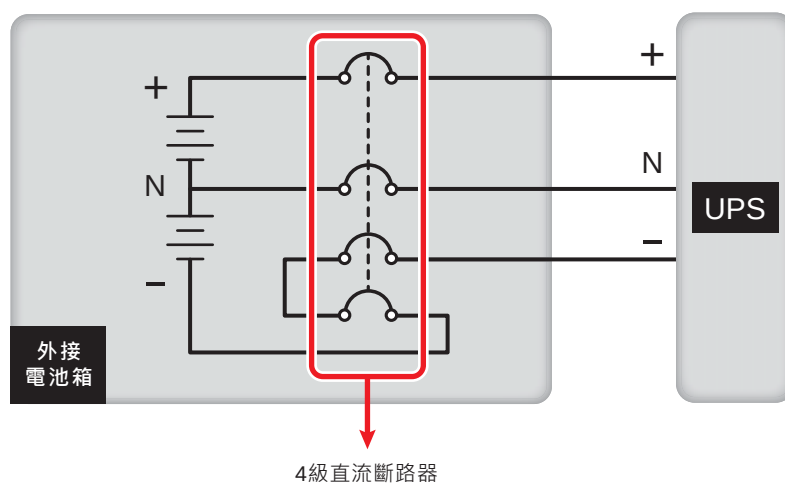
(圖 5-20：安裝 4 極直流斷路器)
