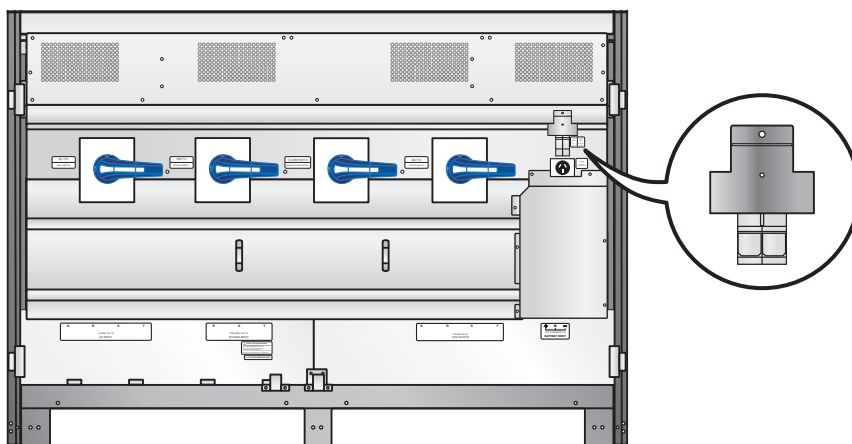
(圖 7-2：接上保險絲座)
