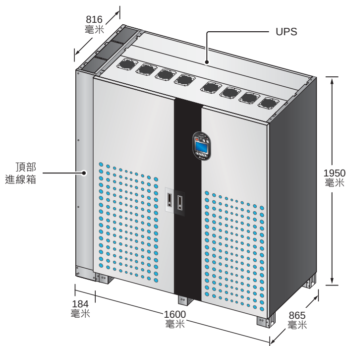
(圖 6-1：外觀和尺寸 (含頂部進線箱))
