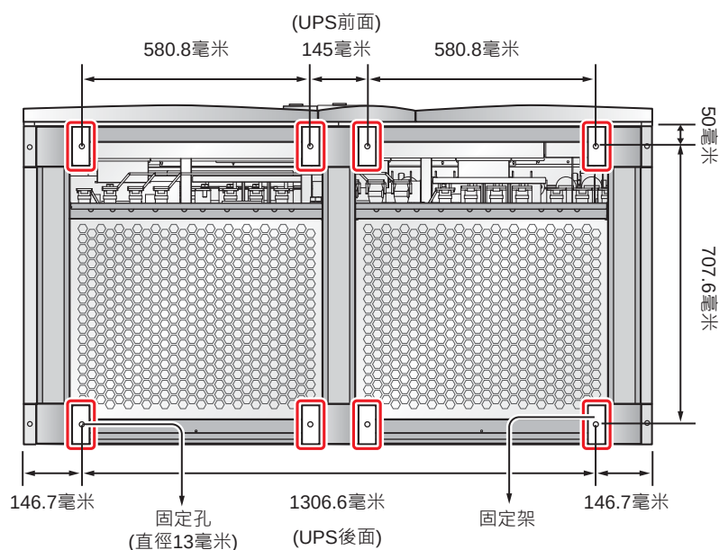
(圖 5-2：孔位圖)
