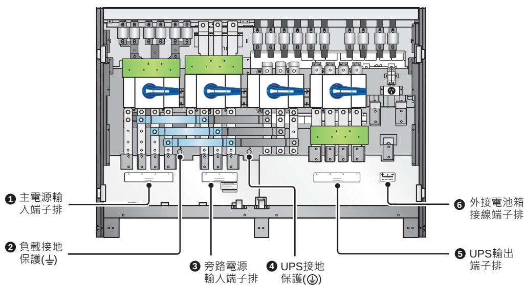
(圖 2-12：配線端子排)
