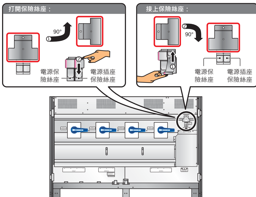
(圖 2-10：打開 / 接上保險絲座)
