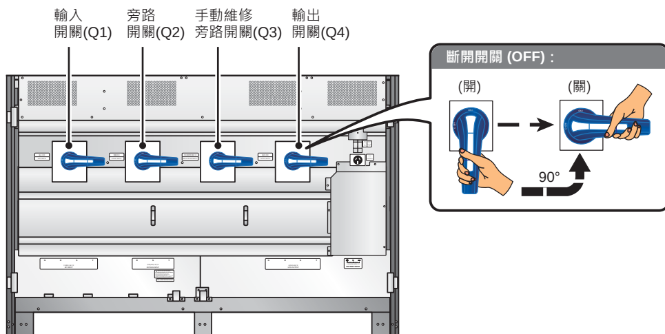
(圖 5-11 : 開關位置與斷開開關)
