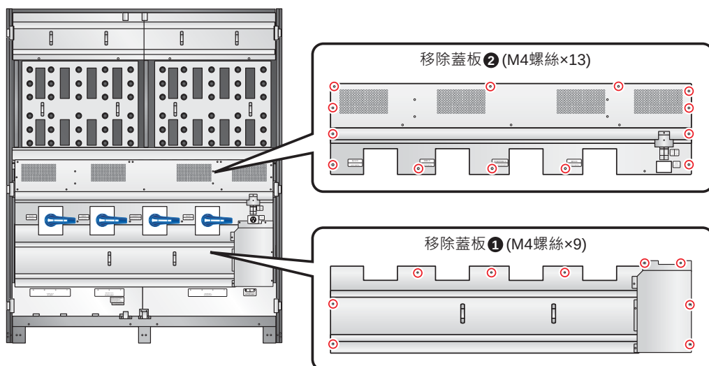
(圖 2-11：蓋板位置)
