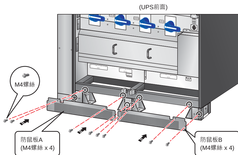
(圖 6-4：在 UPS 前面安裝防鼠板)
