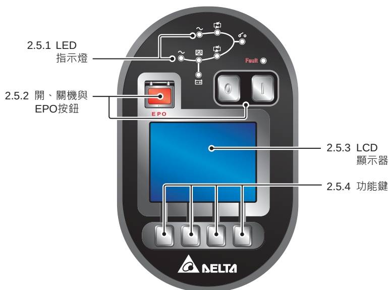
(圖 2-5：控制面板)
