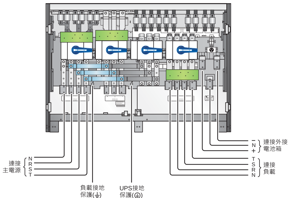
(圖 5-12：單機單迴路輸入 / 輸出配線圖)
