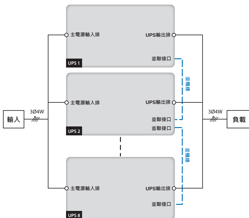
(圖 5-14：並機單迴路輸入 / 輸出配線圖)
