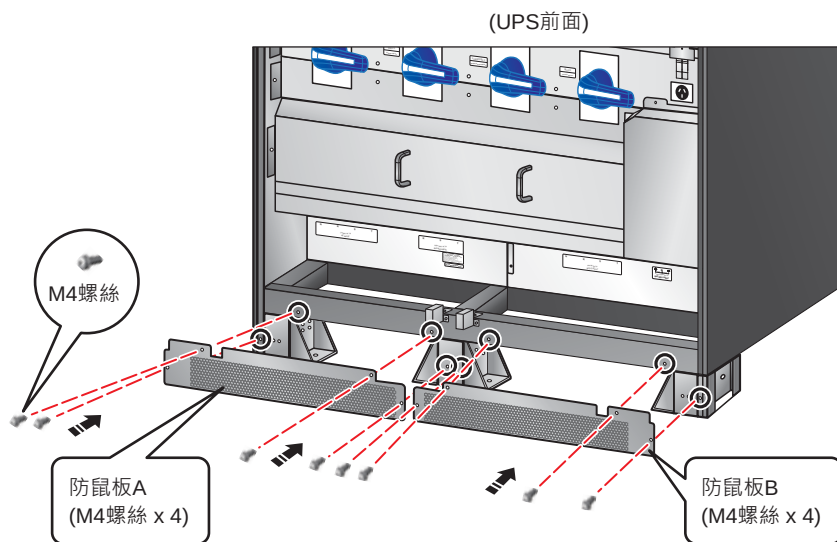
(圖 5-4：在 UPS 前面安裝防鼠板)
