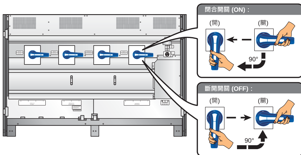
(圖 2-8：閉合 / 斷開開關)
