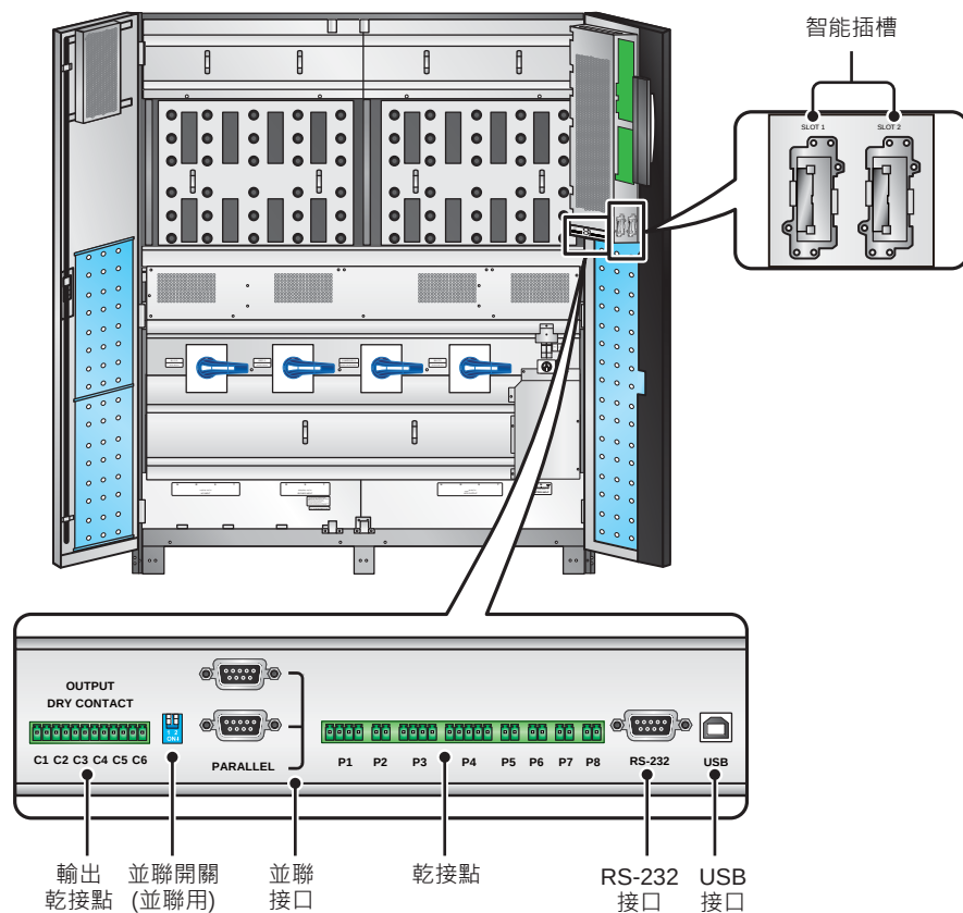
(圖 2-13：通訊界面)
