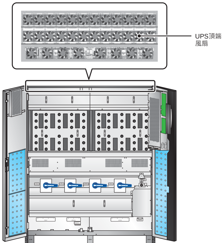
(圖 2-14：風扇位置圖)
