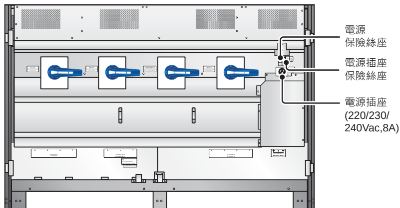
(圖 2-9：保險絲座位置圖)
