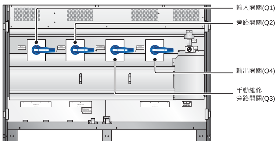
(圖 2-7：輸入與輸出開關)
