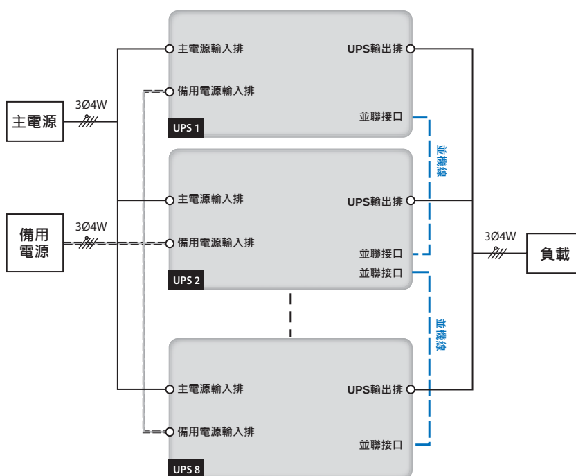
(圖 5-15：並機雙迴路輸入 / 輸出配線圖)
