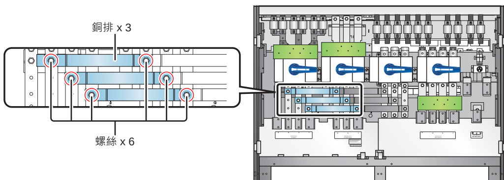
(圖 5-9：六個螺絲和三根銅排位置)
