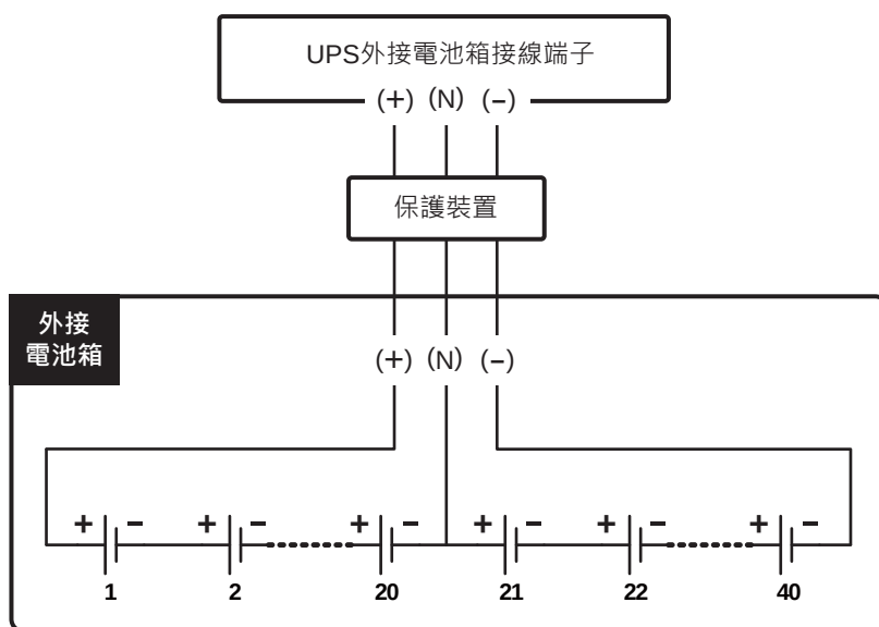
(圖 5-16：連接外接電池箱)
