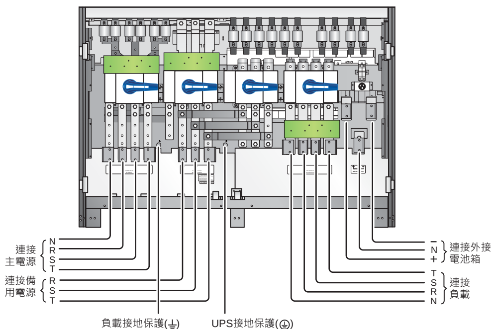
(圖 5-13：單機雙迴路輸入 / 輸出配線圖)
