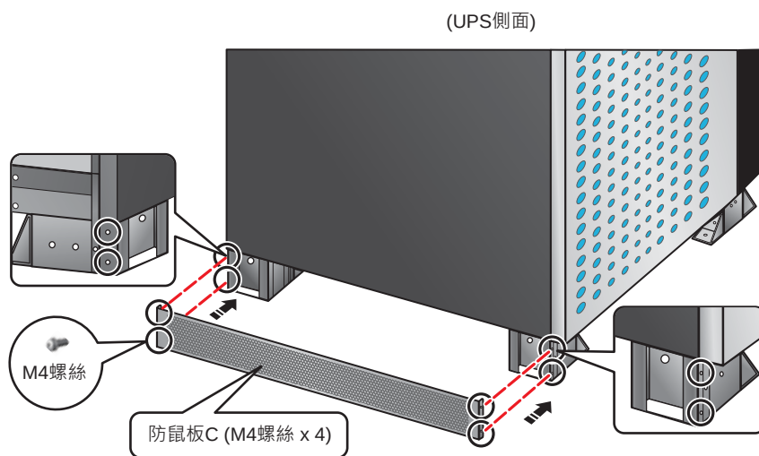
(圖 5-6：在 UPS 側面安裝防鼠板)
