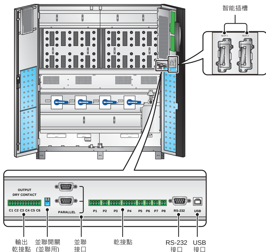
(圖 4-1：通訊界面)
