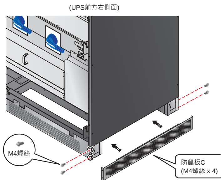
(圖 6-6：在 UPS 前方右側底端安裝防鼠板)
