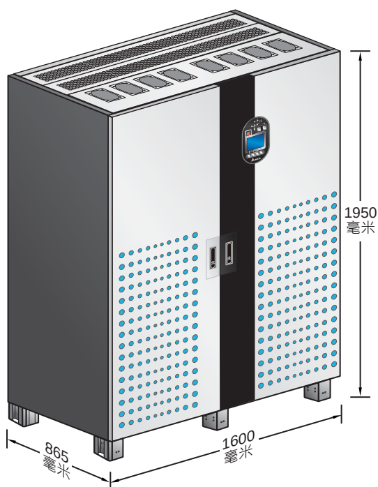
(圖 2-2：尺寸 (不含頂部進線箱))
