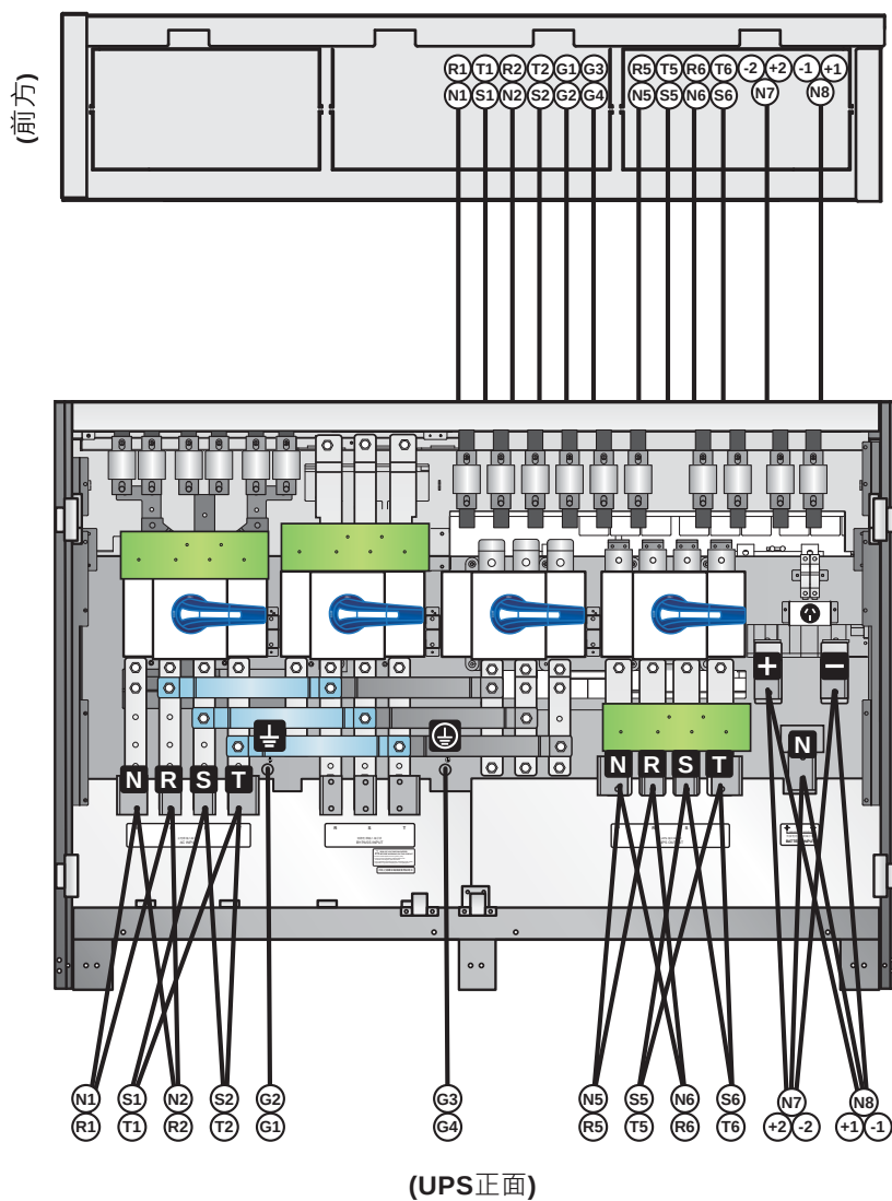
(圖 6-10：建議的走線配線方式_單迴路)
