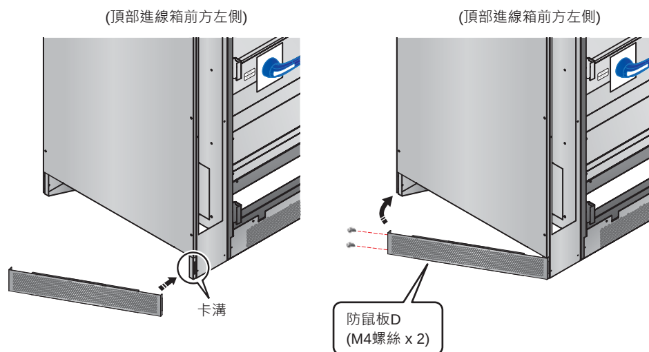
(圖 6-7：在頂部進線箱前方左側安裝防鼠板)
