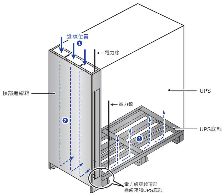
(圖 6-9：進線位置說明圖)
