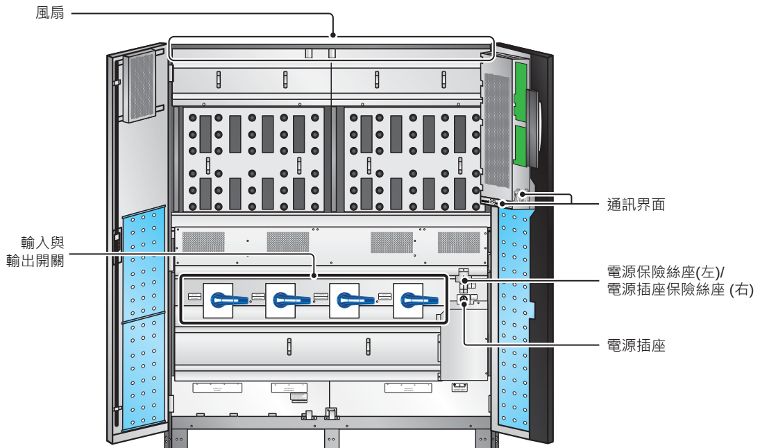
(圖 2-4：機箱內部圖)
