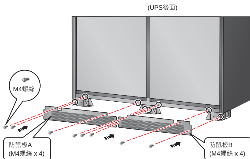
(圖 5-5：在 UPS 後面安裝防鼠板)
