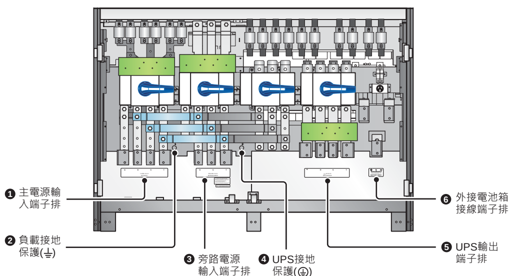
(圖 5-10：配線端子排)
