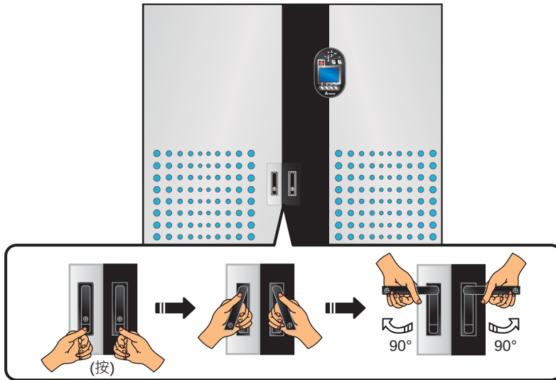
(圖 2-3：前門打開圖)
