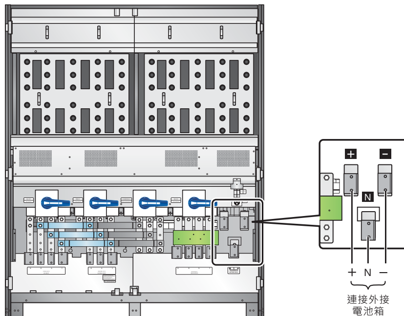
(圖 5-17：外接電池箱配線圖)
