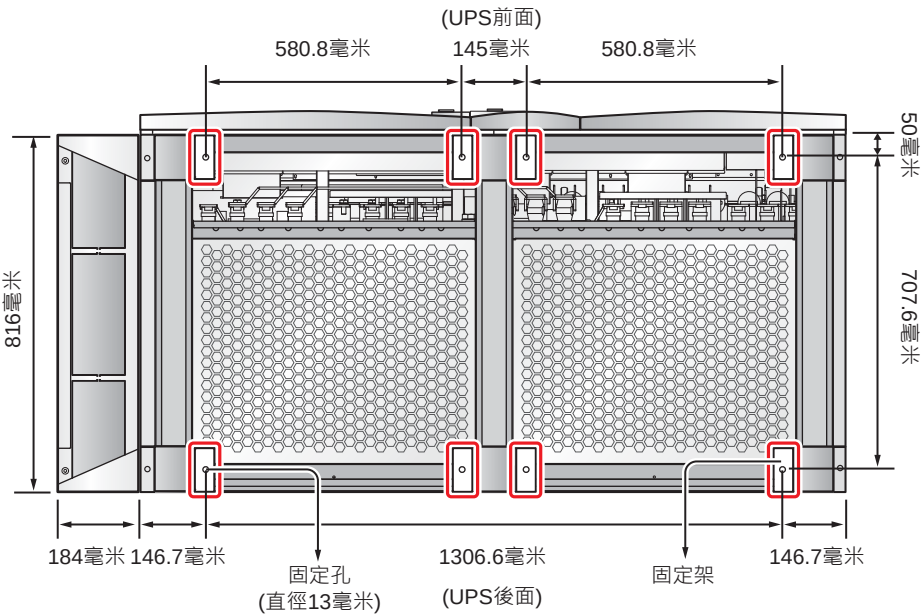
( 圖 6-2：孔位圖 )
