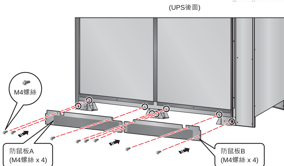
(圖 6-5：在 UPS 後面安裝防鼠板)
