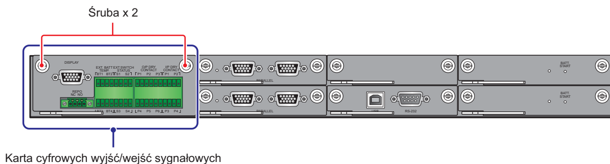
(Rysunek 4-5: Lokalizacja karty cyfrowych wejść/wyjść sygnałowych)
