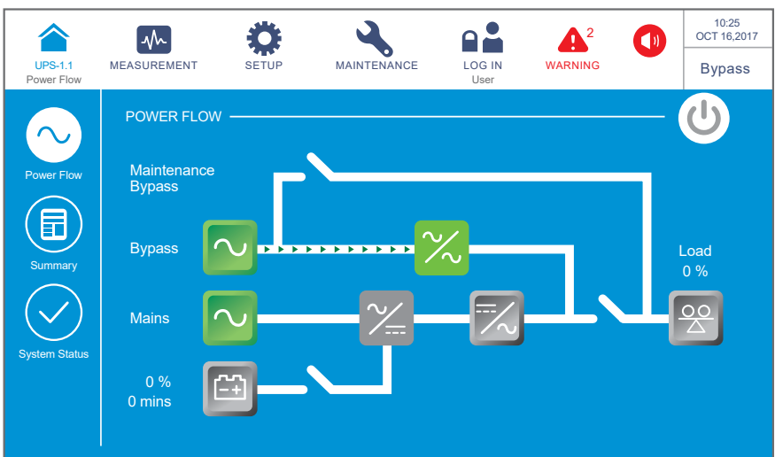
(Rysunek 6-69: Ekran podczas pracy w trybie obejścia (bypass))
