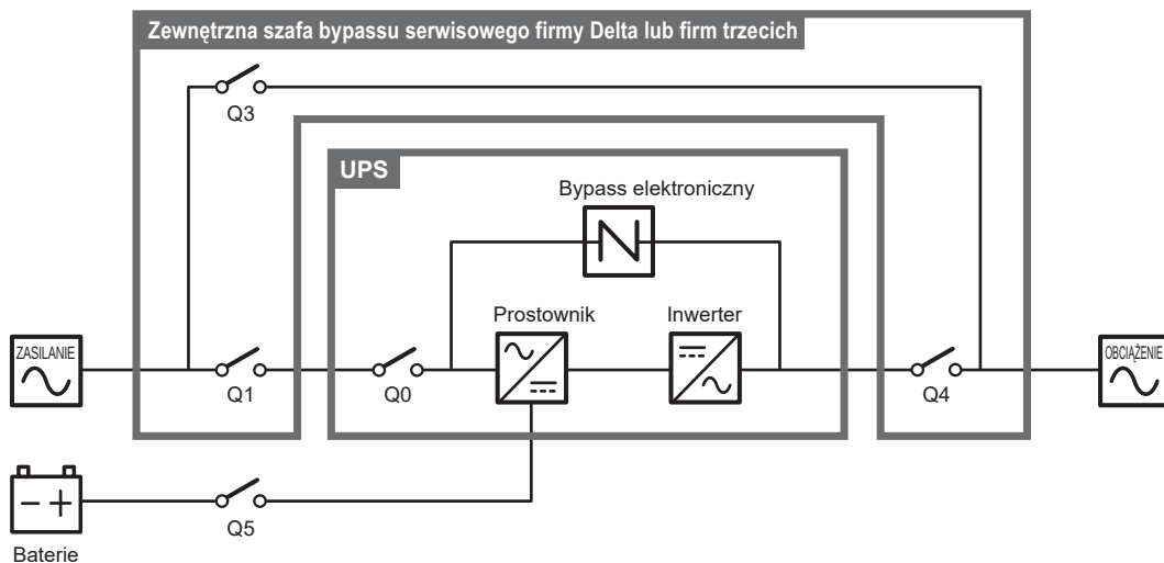
(Rysunek 3-1: Schemat podłączenia zewnętrznej szafy bypassu serwisowego firmy Delta lub firm trzecich przy pojedynczym źródle zasilania)
