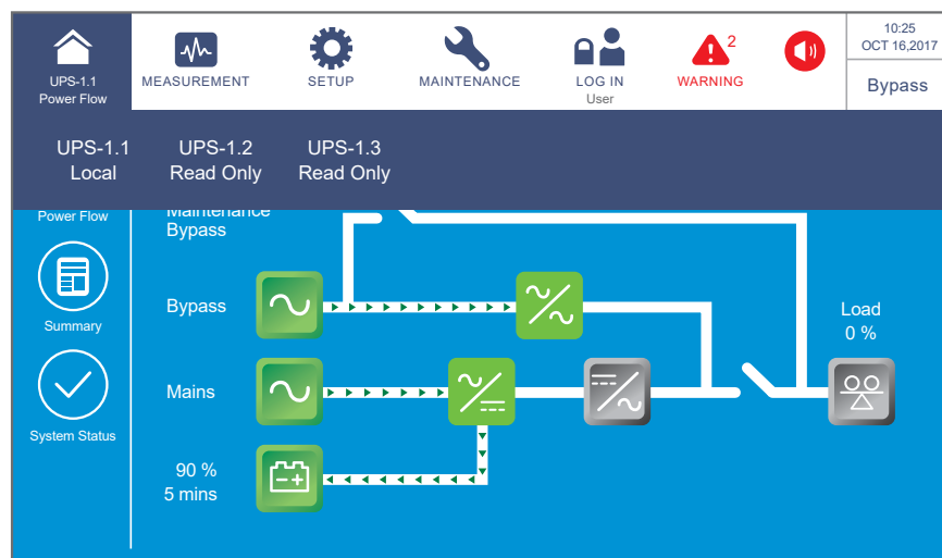
(Rysunek 6-12: Weryfikacja identyfikatorów urządzeń pracujących równolegle)
