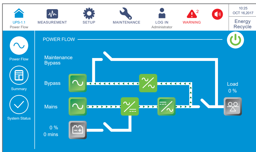
(Rysunek 6-44: Ekran podczas pracy w trybie Recycle Mode)
