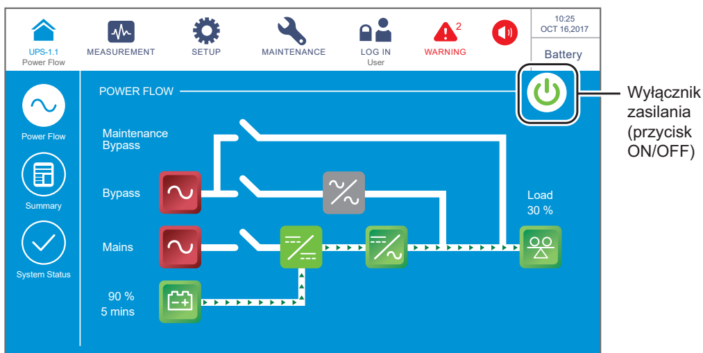
(Rysunek 6-48: Ekran główny w trybie zasilania z baterii – lokalizacja przycisku włącznika zasilania (ON/OFF))
