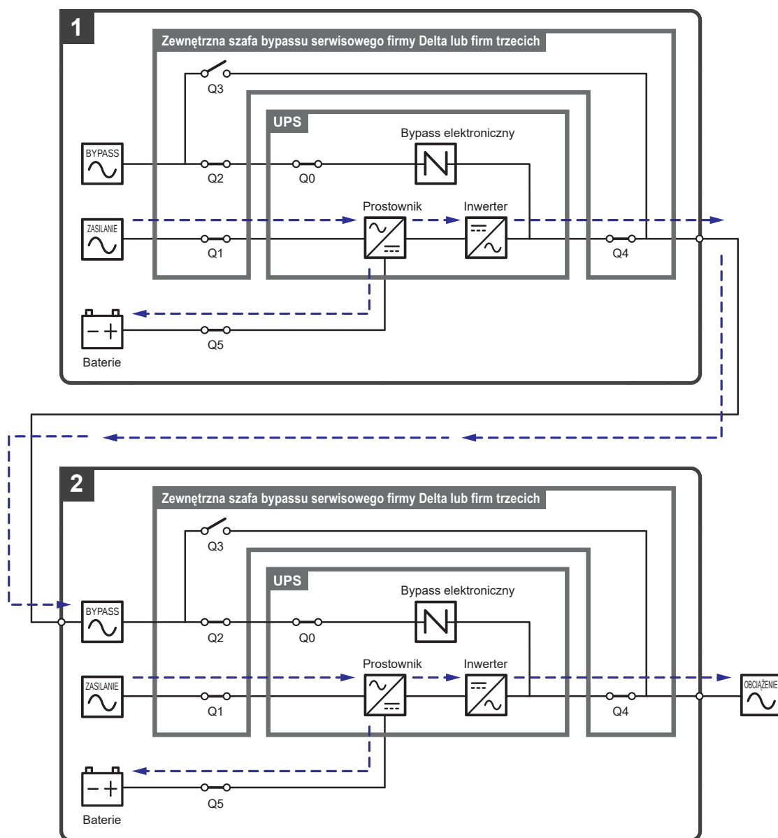
(Rysunek 3-32: Tryb nadmiarowy stałej gotowości (tylko dla podwójnego źródła zasilania i co najmniej dwóch zasilaczy UPS))
