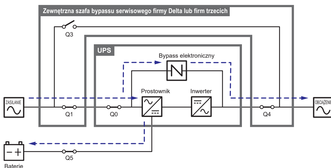
(Rysunek 3-5: Tryb obejścia ( bypass ) (pojedyncze źródło zasilania, pojedynczy UPS))
