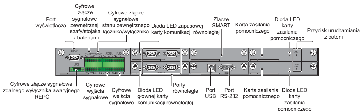
(Rysunek 4-3: Funkcje interfejsów komunikacyjnych)
