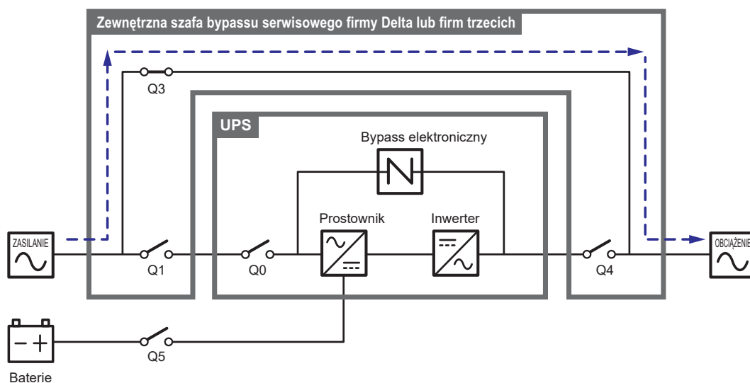
(Rysunek 3-6: Bypass serwisowy (pojedyncze źródło zasilania, pojedynczy UPS))
