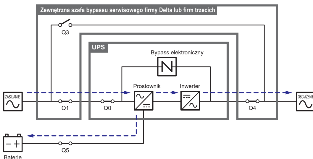
(Rysunek 3-9: Tryb Green (pojedyncze źródło zasilania, pojedynczy UPS))
