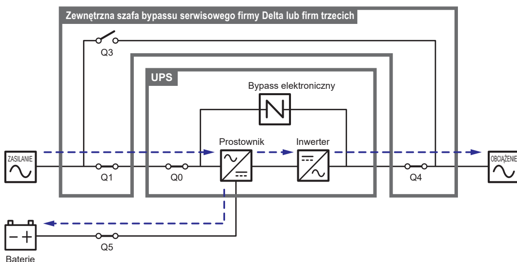
(Rysunek 3-8: Tryb konwersji częstotliwości (pojedyncze źródło zasilania, pojedynczy UPS))
