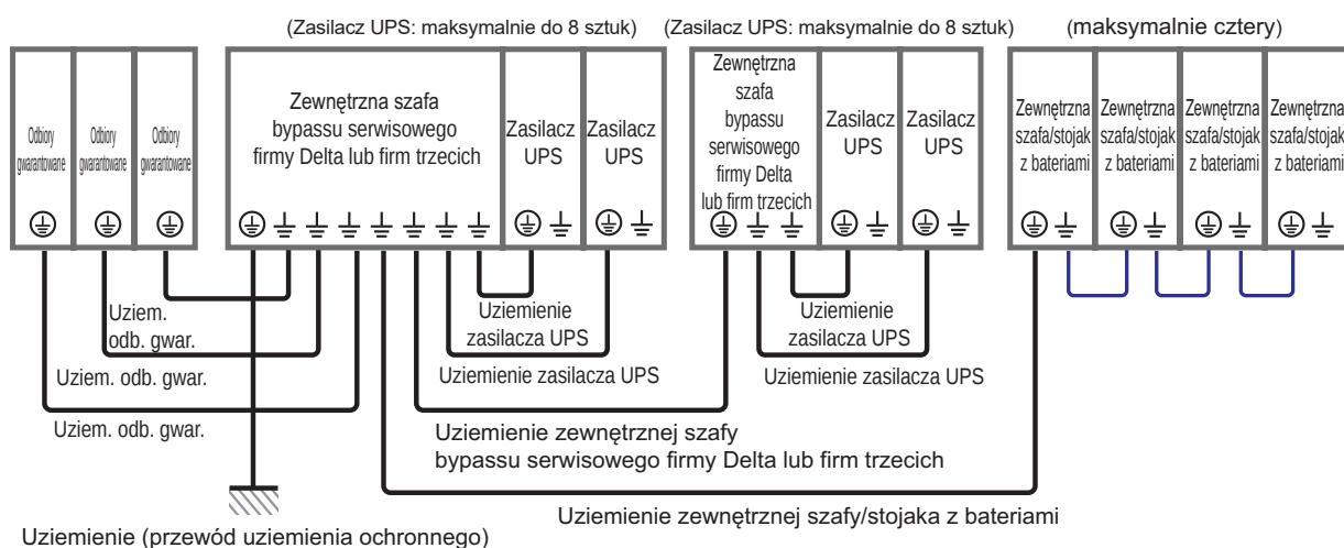
(Rysunek 5-19: Uziemienie jednostek równoległych)
