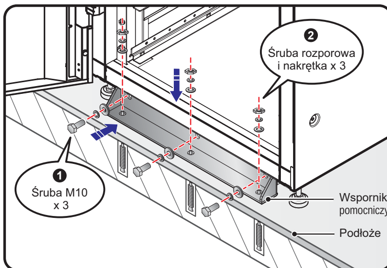
(Rysunek 5-3: Montaż wsporników pomocniczych z przodu zasilacza UPS)
