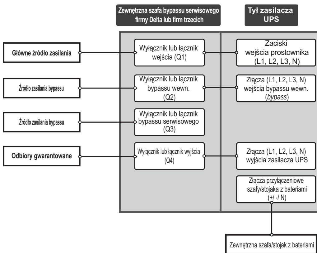
(Rysunek 5-17: Schemat okablowania pojedynczej jednostki dla podwójnego źródła zasilania)
