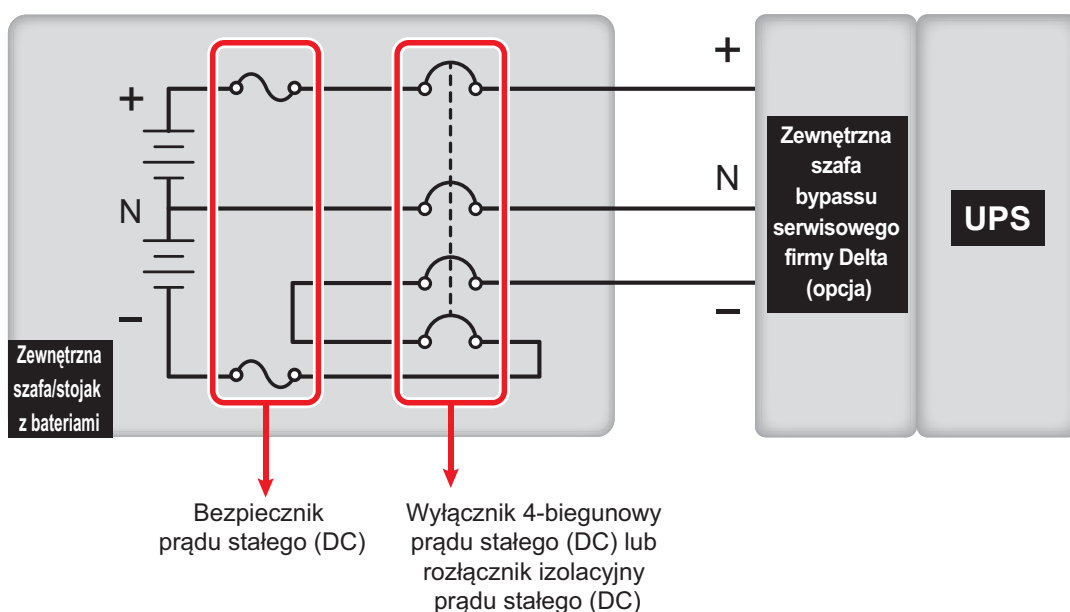
(Rysunek 5-21: Schemat połączenia 4-biegunowego wyłącznika prądu stałego (DC) lub rozłącznika izolacyjnego prądu stałego (DC) połączonego szeregowo z bezpiecznikiem prądu stałego (DC))
