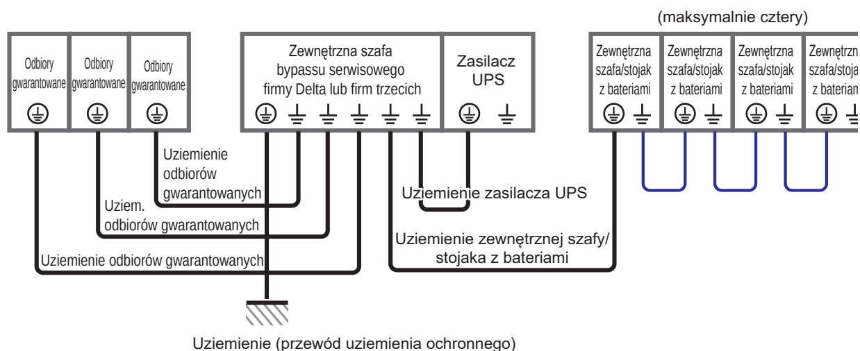
(Rysunek 5-16: Uziemienie pojedynczej jednostki)
