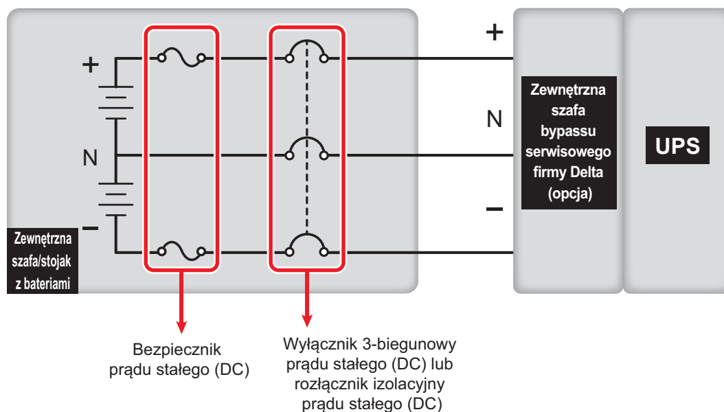
(Rysunek 5-22: Schemat połączenia 3-biegunowego wyłącznika prądu stałego (DC) lub rozłącznika izolacyjnego prądu stałego (DC) połączonych szeregowo z bezpiecznikiem prądu stałego (DC))
