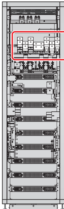
(Widok z tyłu po demontażu panelu tylnego)
