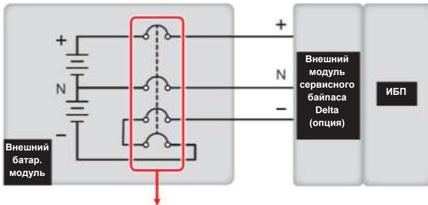
4-полюс. авт. выключатель пост. тока
