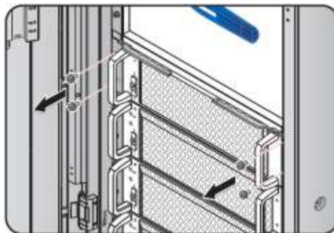
Рисунок 5-33: Снятие 4 винтов
