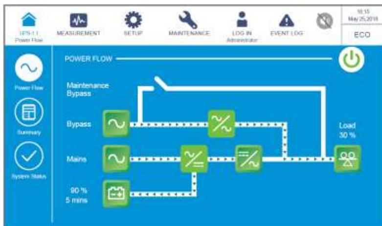
Рисунок 6-26: Экран ECO-режима
