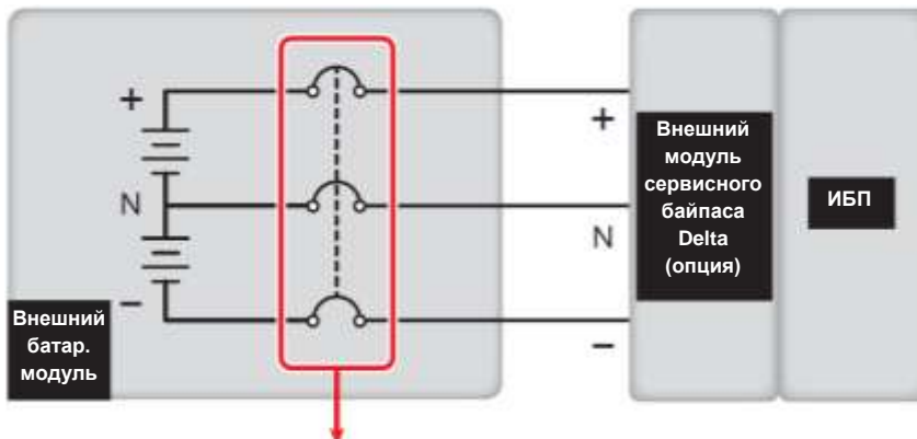
3-полюс. авт. выключатель пост. тока
