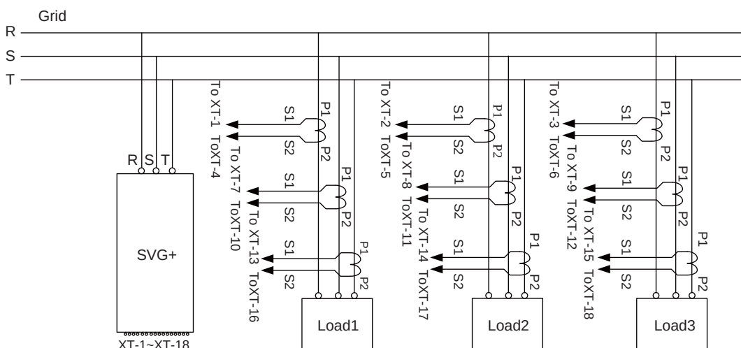
(图 3-10：谐波源比较分散 CT 配线图)
