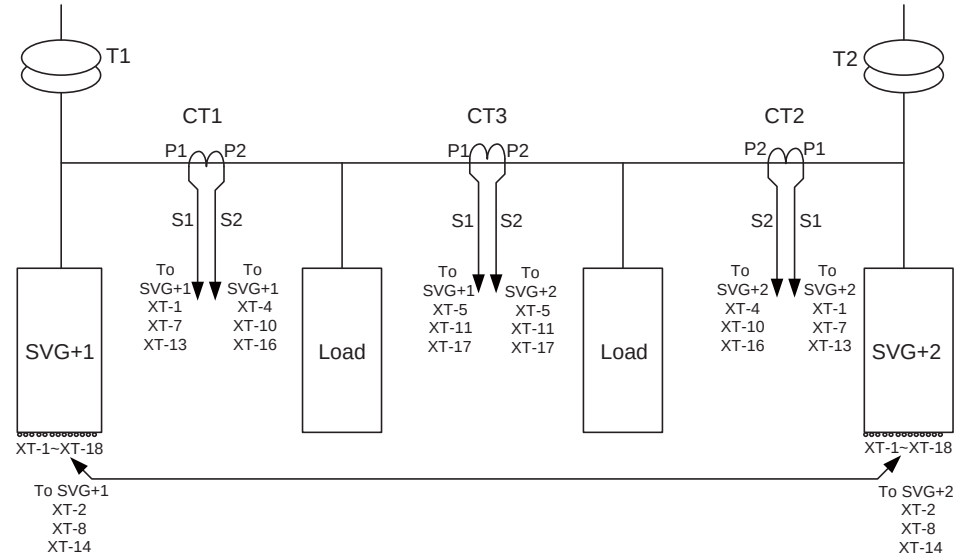
(图 3-13: 两套母线供电 CT 装配图)
