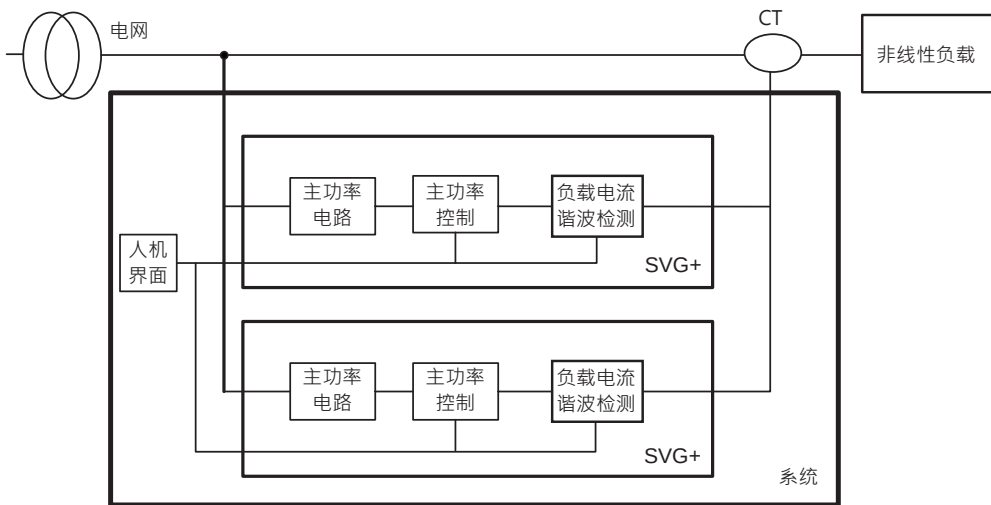
(图 2-1：SVG+ 系统框图)
