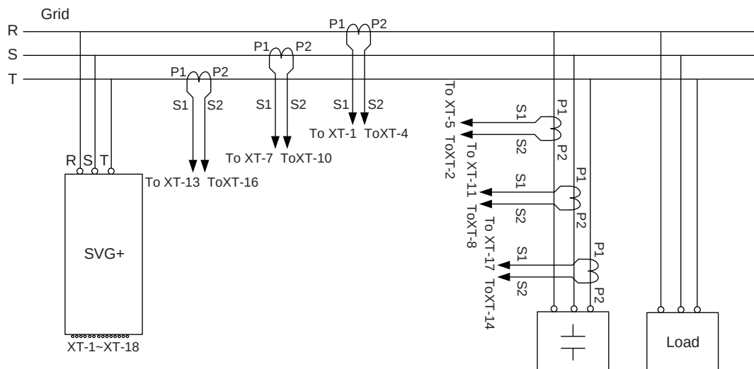
(图 3-11：谐波源侧装有电容补偿柜 CT 配线图)
