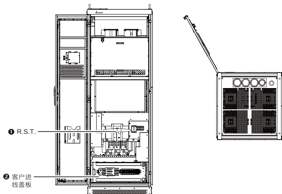
(图 3-3：下进线系统柜结构前视图和底视图)
