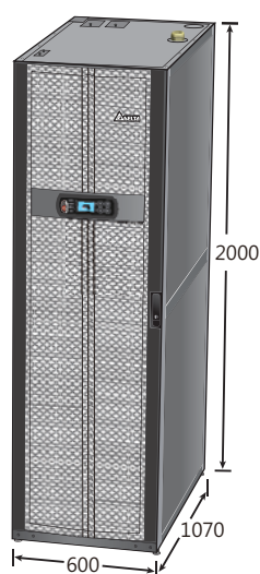
(圖 2-1: 機台整體外觀與尺寸)
