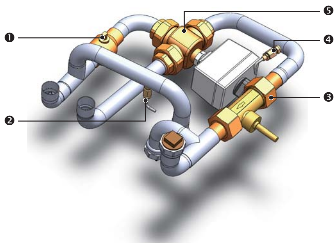
(圖 2-5: 管道主要元件示意圖)
