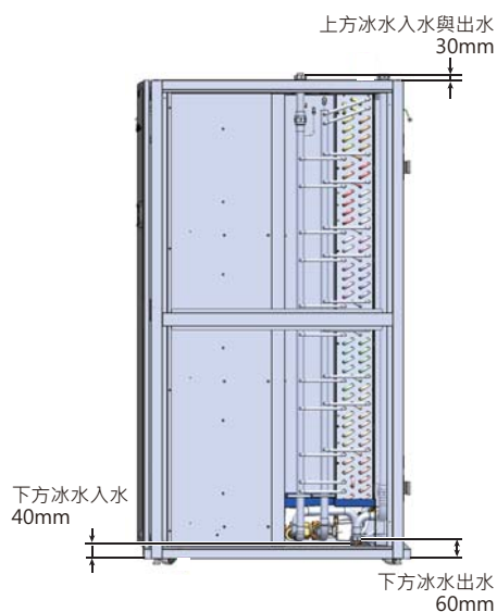
(圖 3-7：上下配管位置尺寸圖)
