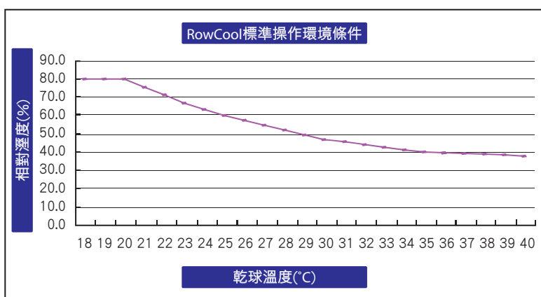
(圖 4-2：標準操作環境條件)
