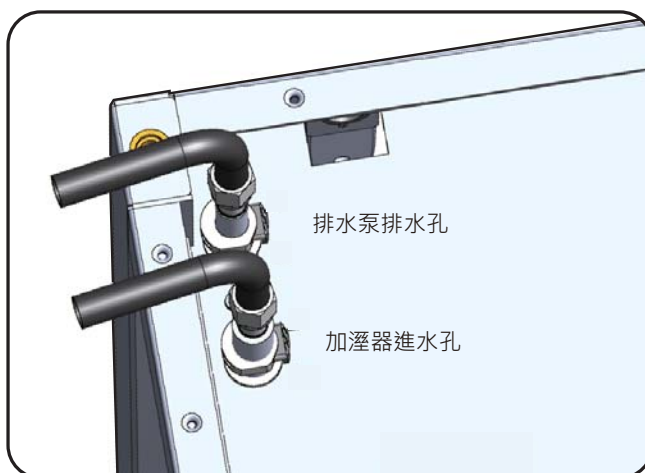
(圖 3-10: 排水泵排水與加溼器進水接管示意圖)
