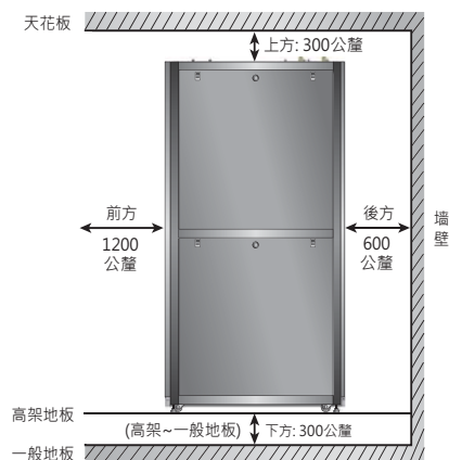
(圖 3-1：淨空範圍)
