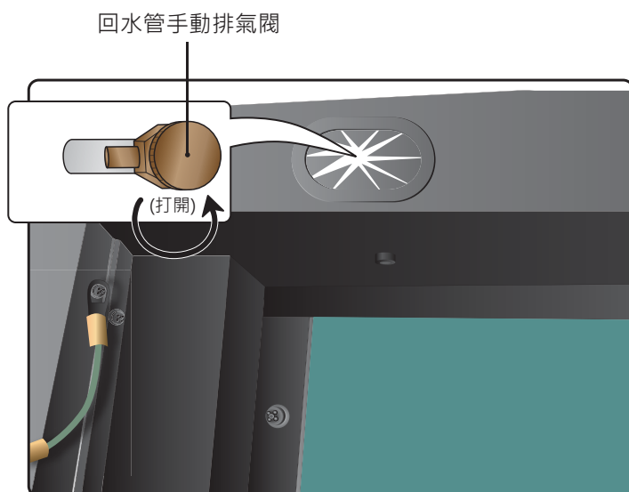
(圖 4-3: 打開回水管手動排氣閥)
