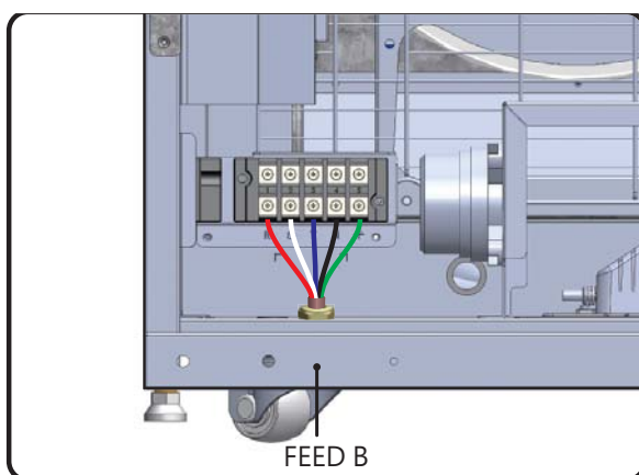
(圖 3-16: 入電接線位置與接線方式)
