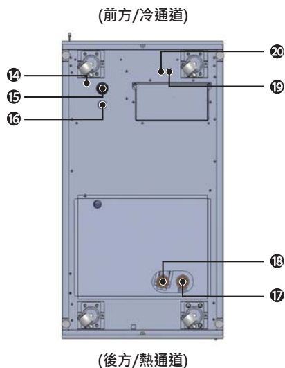
(圖 2-3: 底視元件示意圖)
