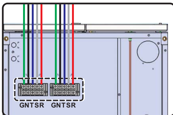
(圖 3-13: 安裝電源線)
