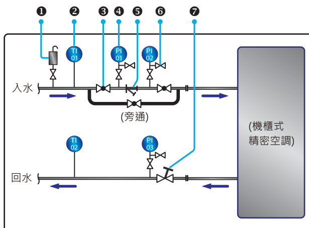
(圖 3-9：建議外部配管)
