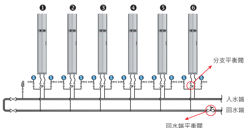
(圖 4-4: 水量平衡)
