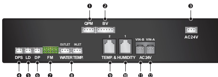
(圖 3-18：控制盒背面)
