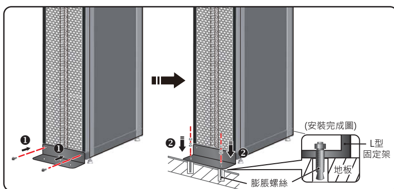
(圖 3-5：安裝 L 型固定架)
