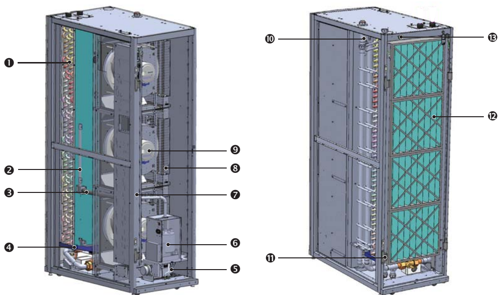
(圖 2-4: 內部元件示意圖)
