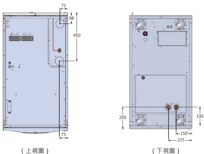
(圖 3-8：上下配管孔徑位置) (單位：mm)
