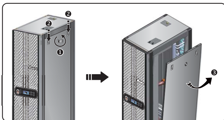
(圖 3-6：移除側板)
