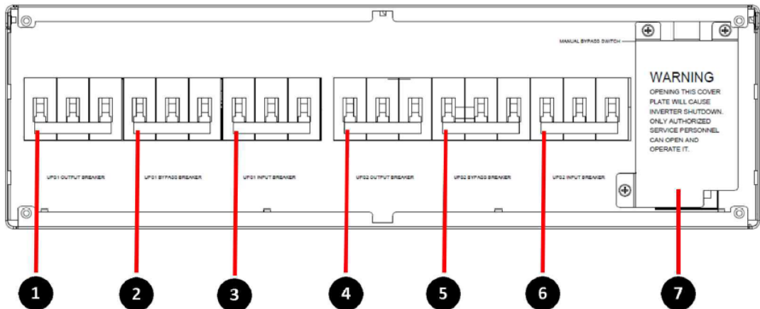
Рис. 4-3. Внутренняя передняя панель БРП
