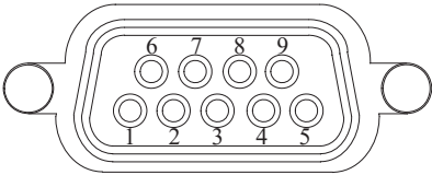
图 8-1 脚位配置图
