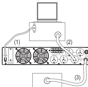
图 3-3.7 UPS 连接 (3 KVA)
