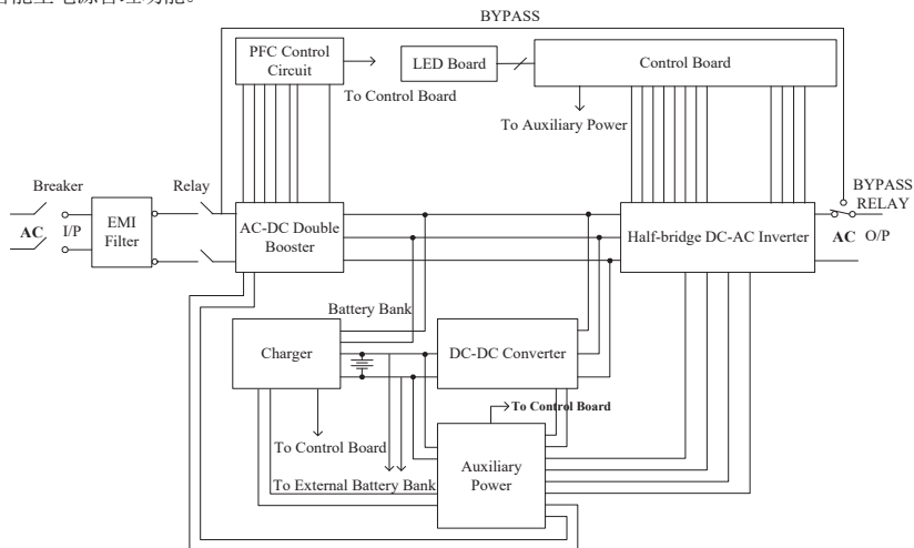
图 2-1.1 UPS 系统方块图
