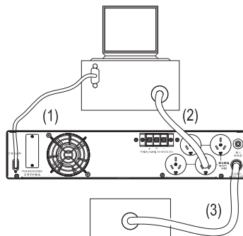
图 3-3.5 UPS 连接 (1KVA 延机)
