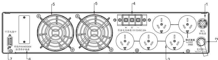
图 2-6.3 2KVA 机种的后背板
