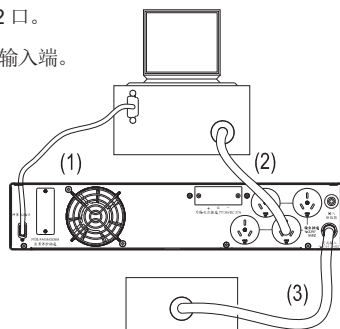
图 3-3.5 UPS 连接 (1KVA 标机)
