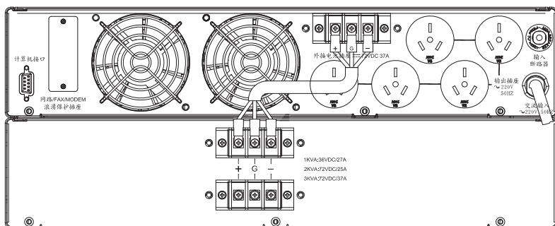
图 3-3.4 UPS 外接电池箱(3 KVA)
