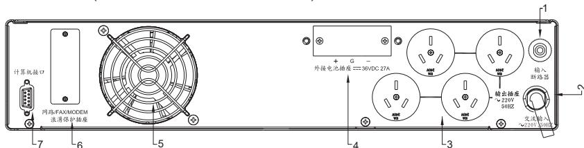
图 2-6.1 1KVA 标机机种的后背板
