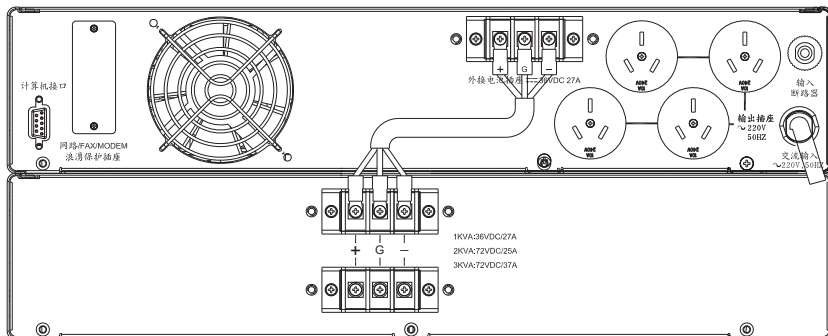
图 3-3.2 UPS 外接电池箱(1 KVA)
