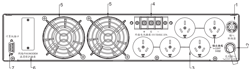
图 2-6.4 3KVA 机种的后背板
