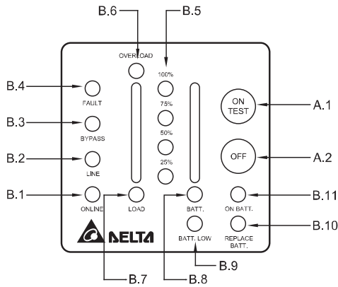
图 2-5.1 操作面板
