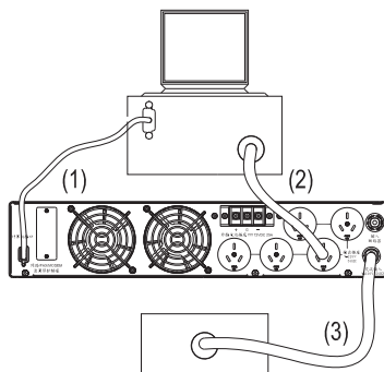
图 3-3.6 UPS 连接 (2 KVA)
