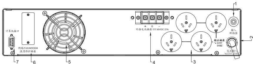
图 2-6.2 1KVA 延机机种的后背板
