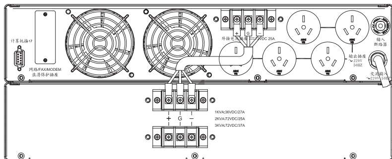
图 3-3.3 UPS 外接电池箱(2 KVA)
