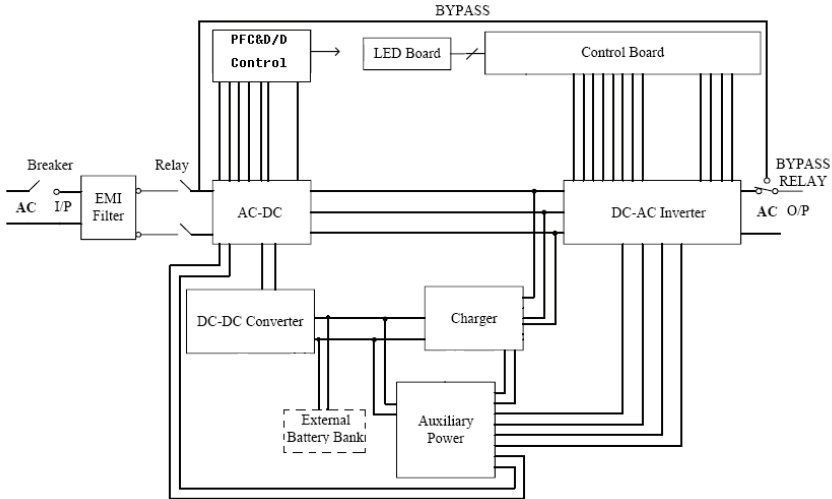
图表 1 2-1.1 UPS 系统方块图
