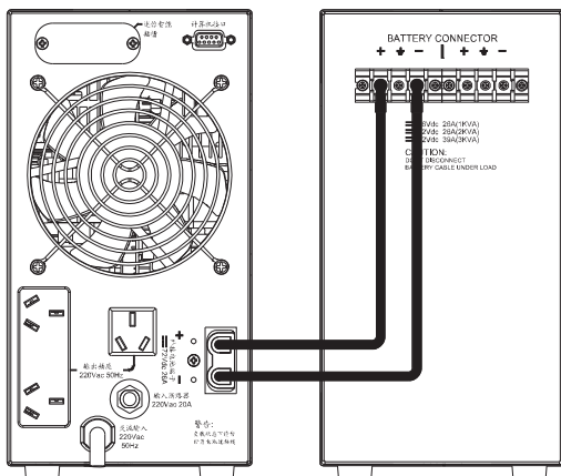
图 3-3.3 UPS 外接电池箱(2/3KVA)
