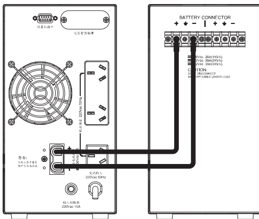
图 3-3.2 UPS 外接电池箱(1KVA)
