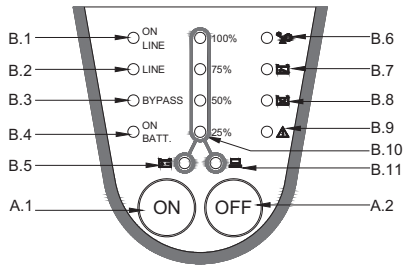
2-5.1 1-3KVA 机种操作面板
