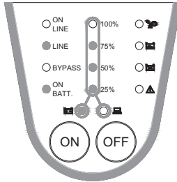
4-3 UPS 自我测试
