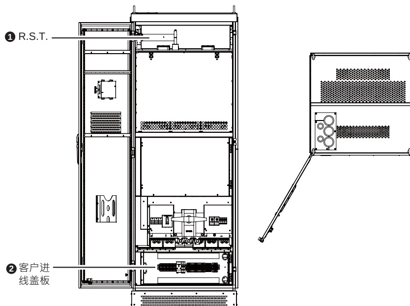
(图 3-4 : 500/ 600kVar 上进线系统柜结构前视图和顶视图)
