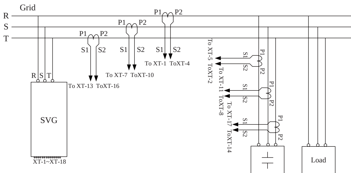
(图 3-14：负载侧装有电容补偿柜 CT 配线图)
