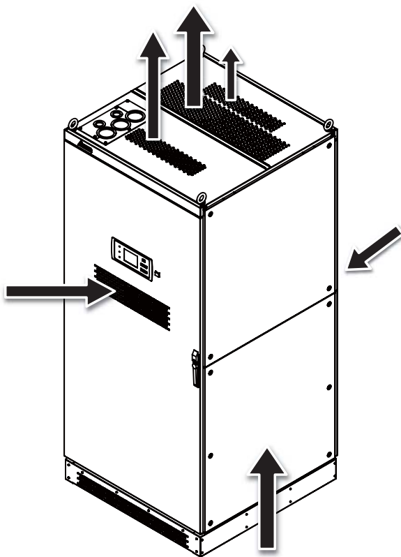
(图 3-1：SVG 系统进出风口示意图)
