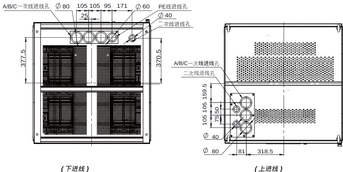
(图 3-10 : 500/ 600kVar 上下进线机型进线位置图)
