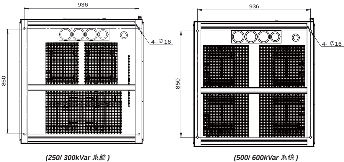
(图 3-8：系统机柜底部定位孔)
