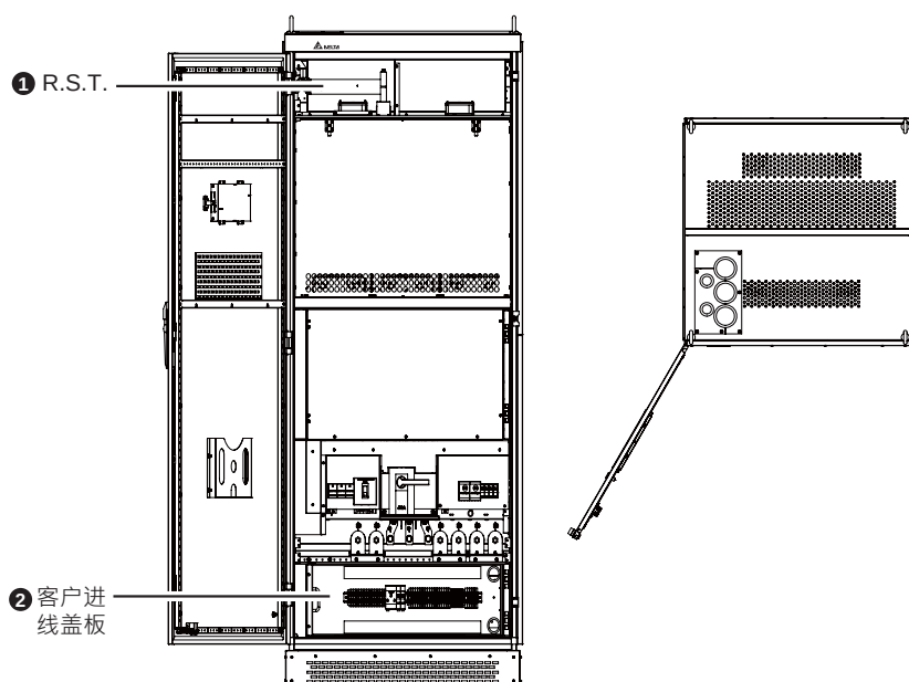
(图 3-2 : 250/ 300kVar 上进线系统柜结构前视图和顶视图)
