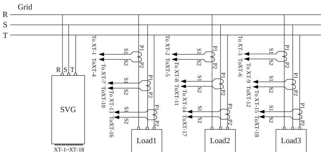
(图 3-13：负载比较分散 CT 配线图)
