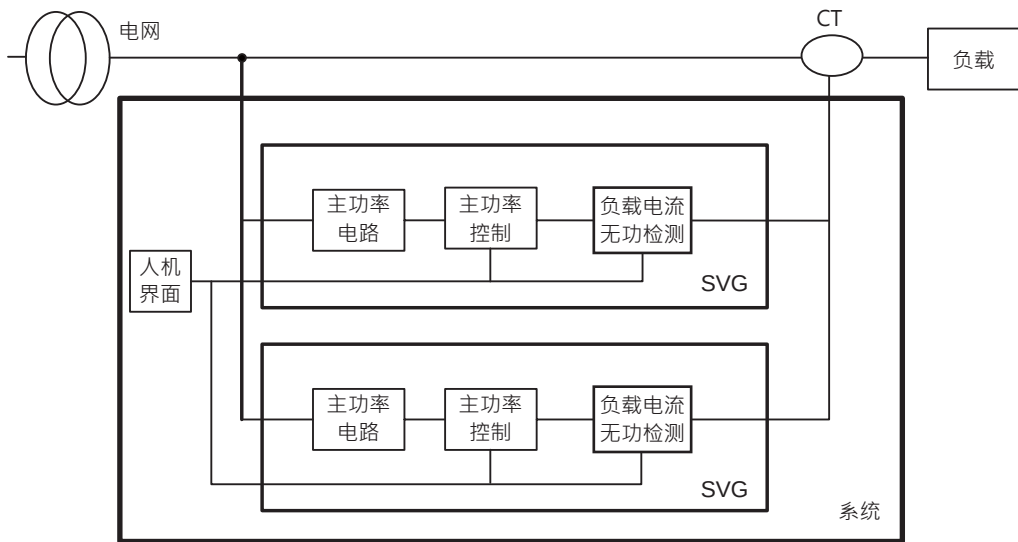
( 图 2-1 : SVG 系统框图 )
