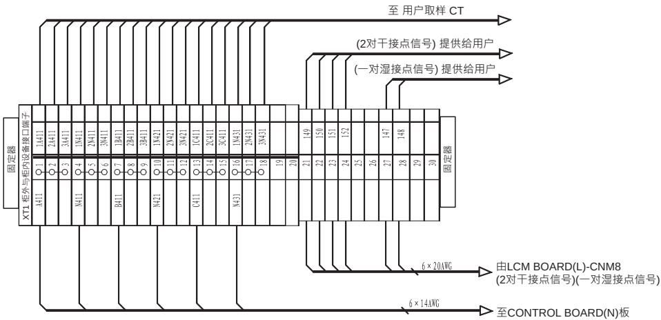
(图 3-11 : CT 及干湿节点接线图)
