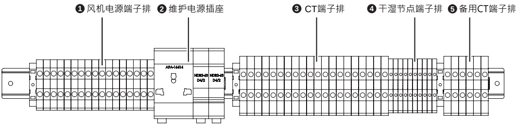
(图 3-6：客户进线面板)
