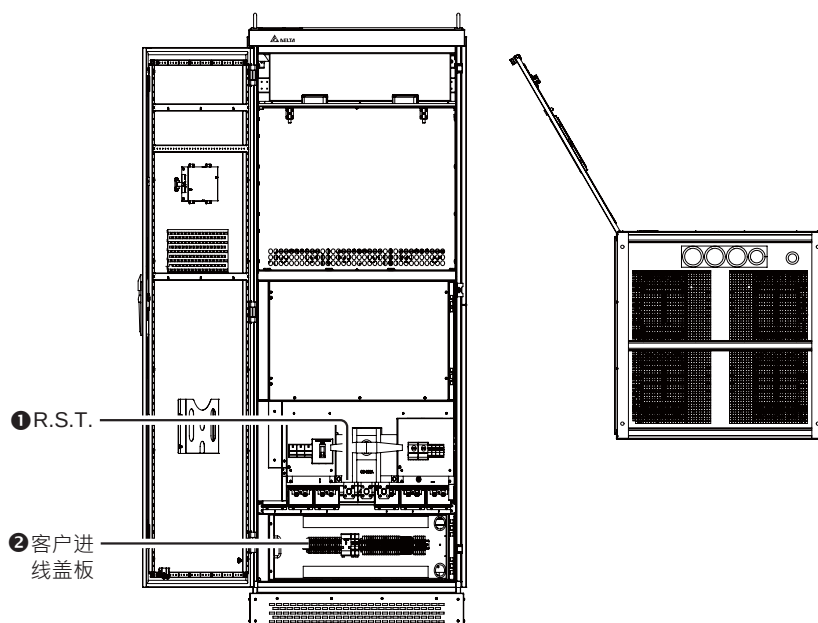
(图 3-5: 500/ 600kVar 下进线系统柜结构前视图和底视图)
