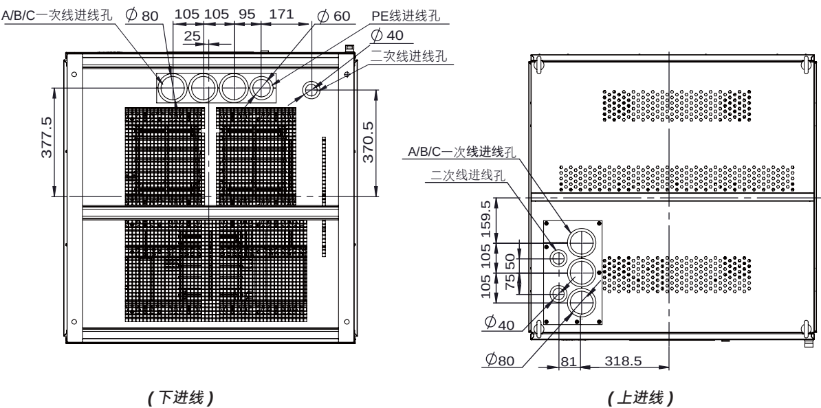
(图 3-9：250/300kVar 上下进线机型电缆进线位置图)
